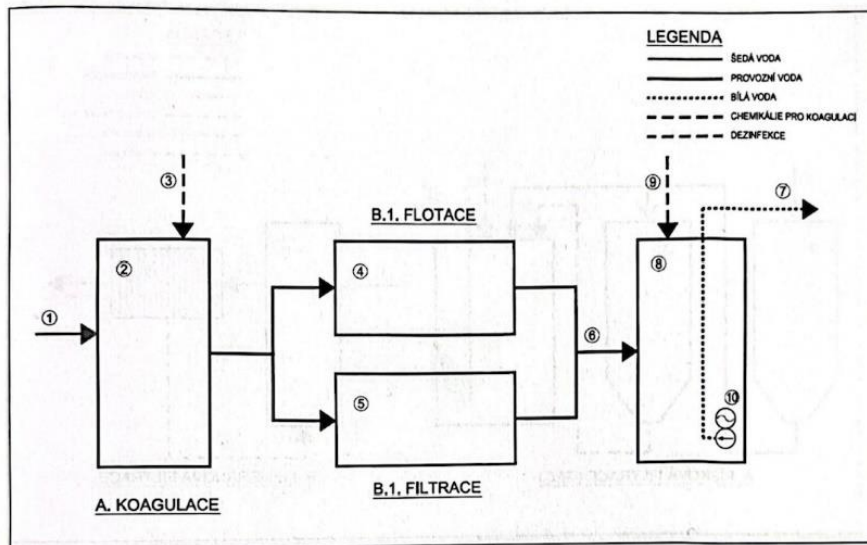
Obrázek 12: Schéma chemického čištění (ČSN 75 6780).
