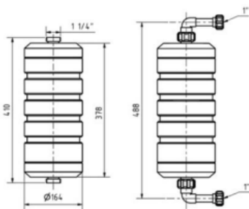
Obr. 4 Membránová patry
