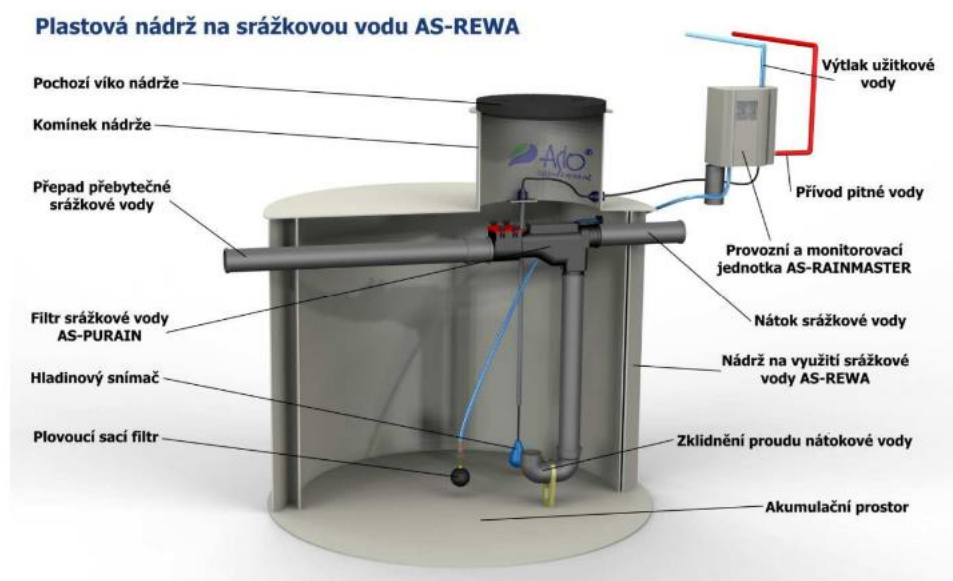
Obrázek 34: Plastová nádrž na srážkovou vodu AS-REWA (ASIO ©2021).
