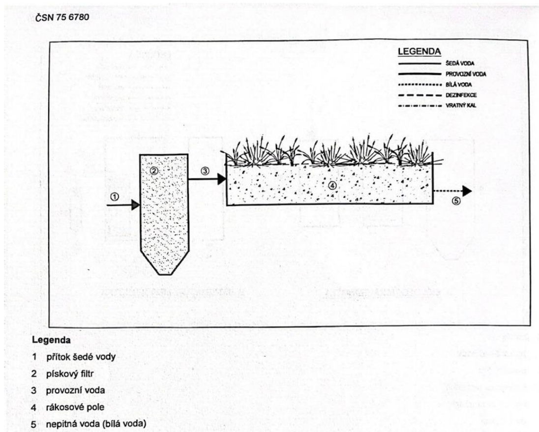
Obrázek 15: Technologické schéma čištění přírodním způsobem (ČSN 75 6780).
