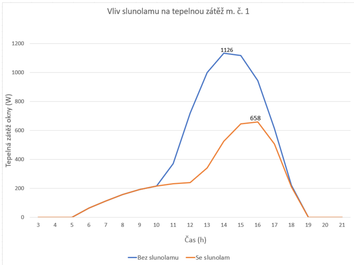
Graf 7 Vliv slunolamu na tepelnou zátěž okny m.č. 1
