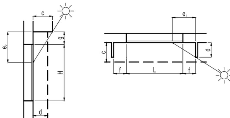
Obr. 7 Oslunění oken
