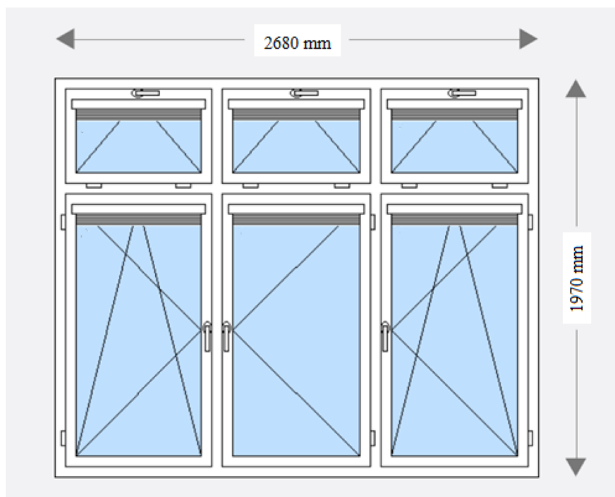
Obr. 22 Náhled oken v konfiguratoru včetně žaluzií pro místnost č. 3
