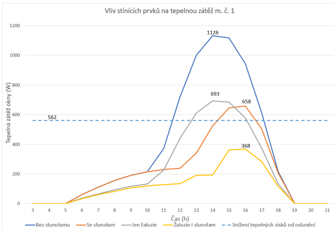
Graf 8 Vliv stínících prvků na tepelnou zátěž okny m.č. 1
