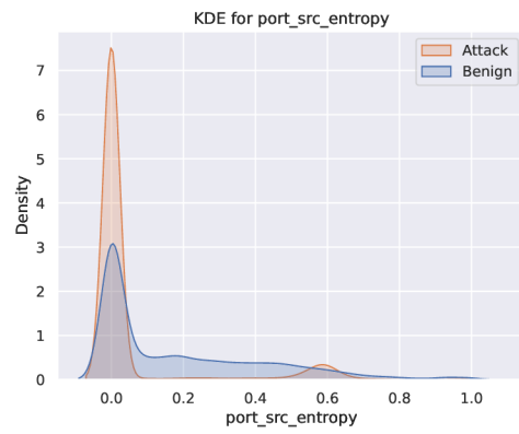
(d) Source port entropy density.
