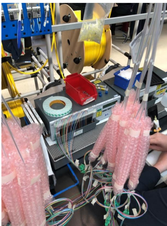
Obr. 4.6 Bublíková fólie na přechodu vlákno-sekundární ochrana [26].
