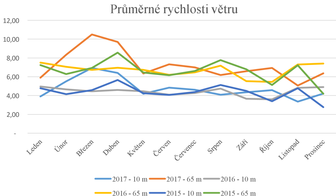
Graf. 5 - Graf naměřených a vypočítaných hodnot průměrných rychlostí větru
