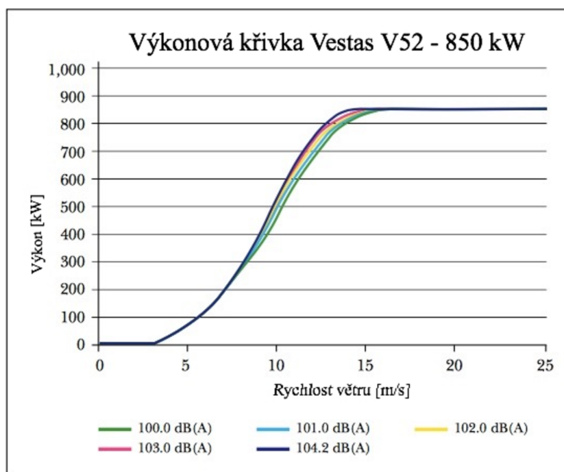
Graf. 4 - Výkonová křivka elektrárny Vestas V52 - 850 kW [17]
