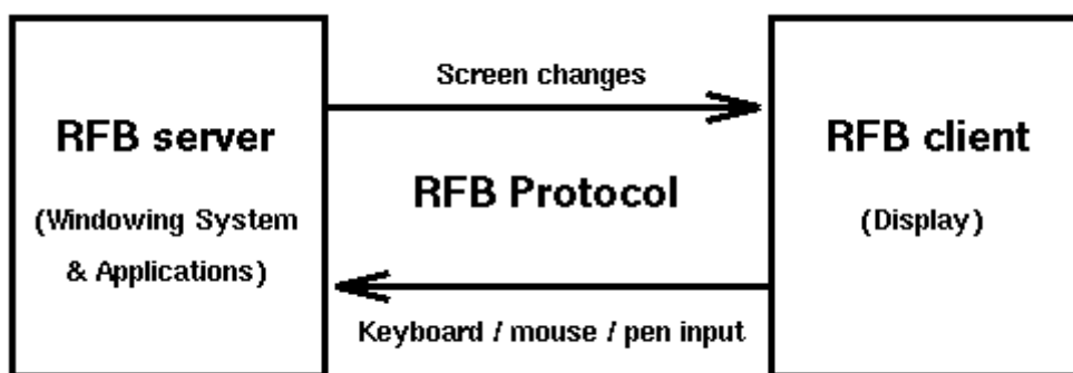
Obrázek 11: RFB protokol [32]
