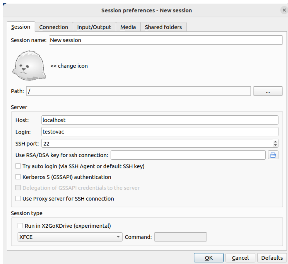
Obrázek 17: X2Go klient [10]
