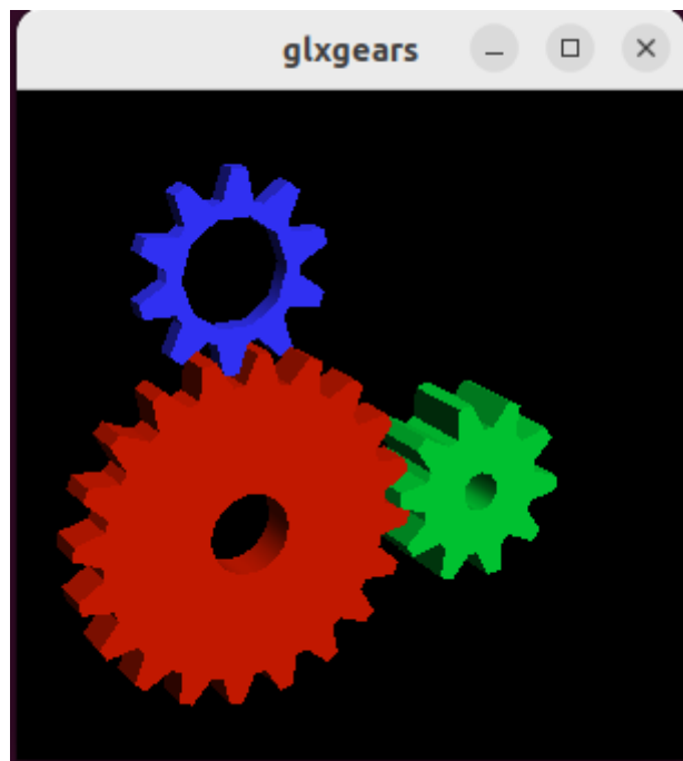
Obrázek 5: Glxgears [10]
