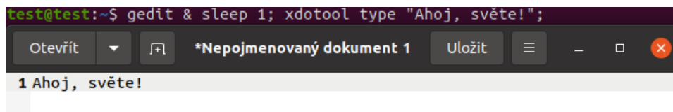
Obrázek 4: Xdotool [10]
