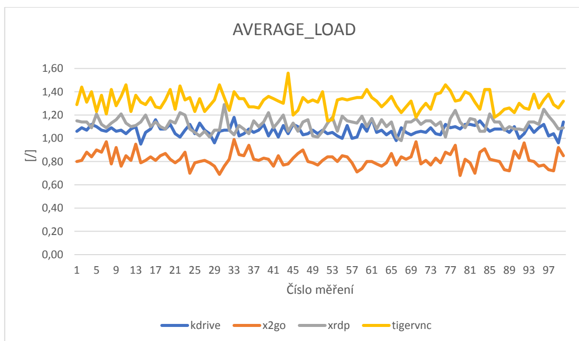
Obrázek 45: Průměrný load [10]
