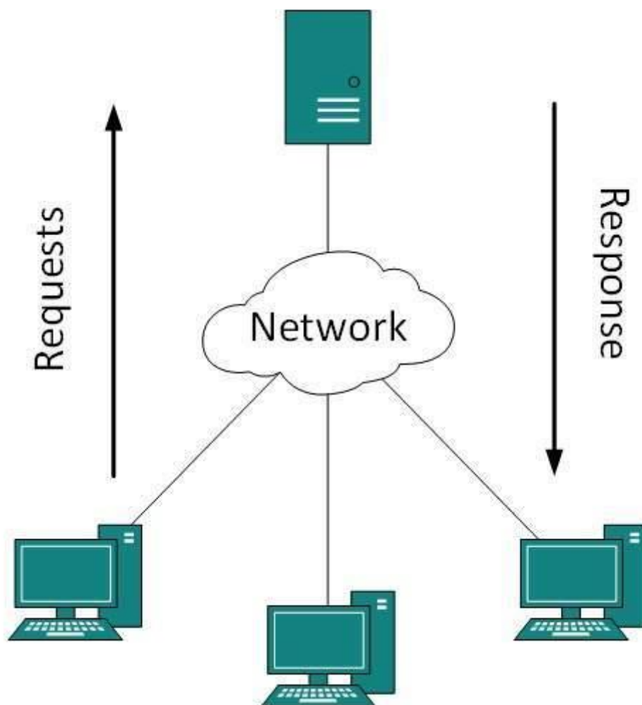
Obrázek 9: Model klient-server [19]
