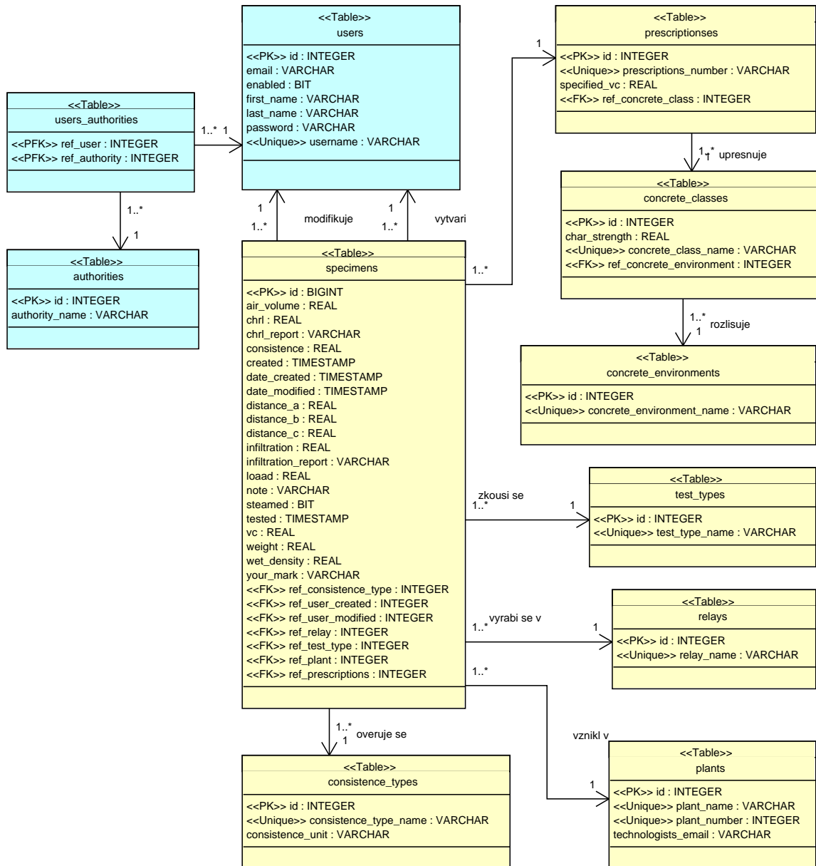
Obrázek 5.2: ER-diagram databáze
