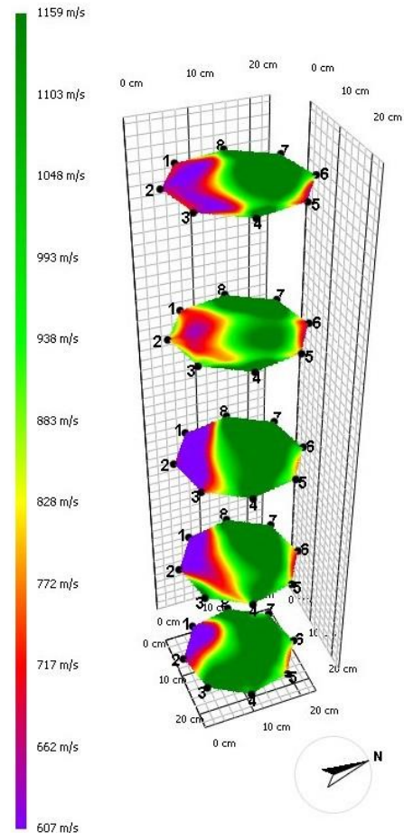
Obrázek 48: Tomograf prvku z měření ultrazvukem (Zdroj: Autor práce)
