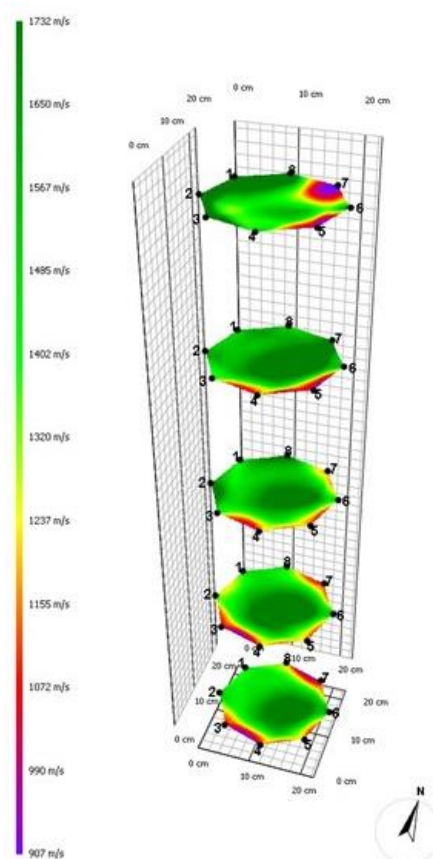
Obrázek 53: Tomograf prvku z měření ultrazvukem (Zdroj: Autor práce)
