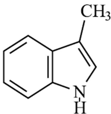
Obrázek 2: Skatol (Haugen 2010)
