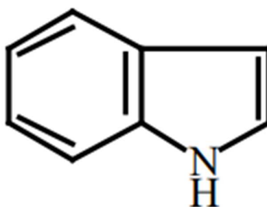
Obrázek 2: Indol (Gribble 2003)
