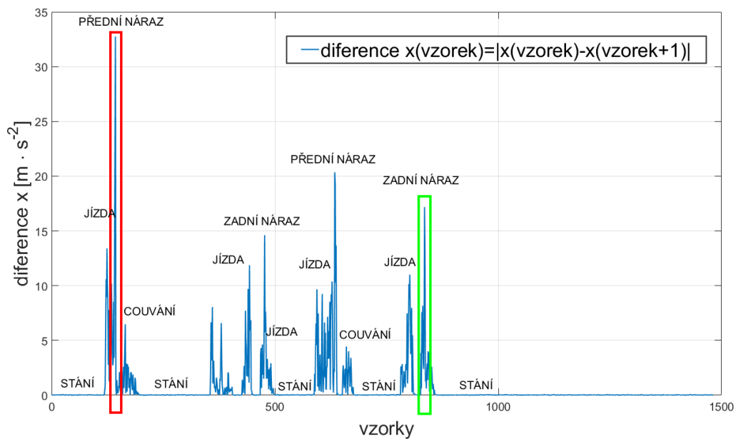
Obr. 3.20: Akvizice dat při nárazu; difference v ose x ze záznamu s více nárazy
