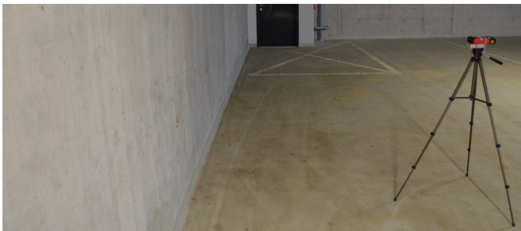
Obr. 10.1: Instalace při měření vzdálenosti 2m pomocí Tagu IMU v4r7 s implementovaným laserovým senzorem VL53L1X
