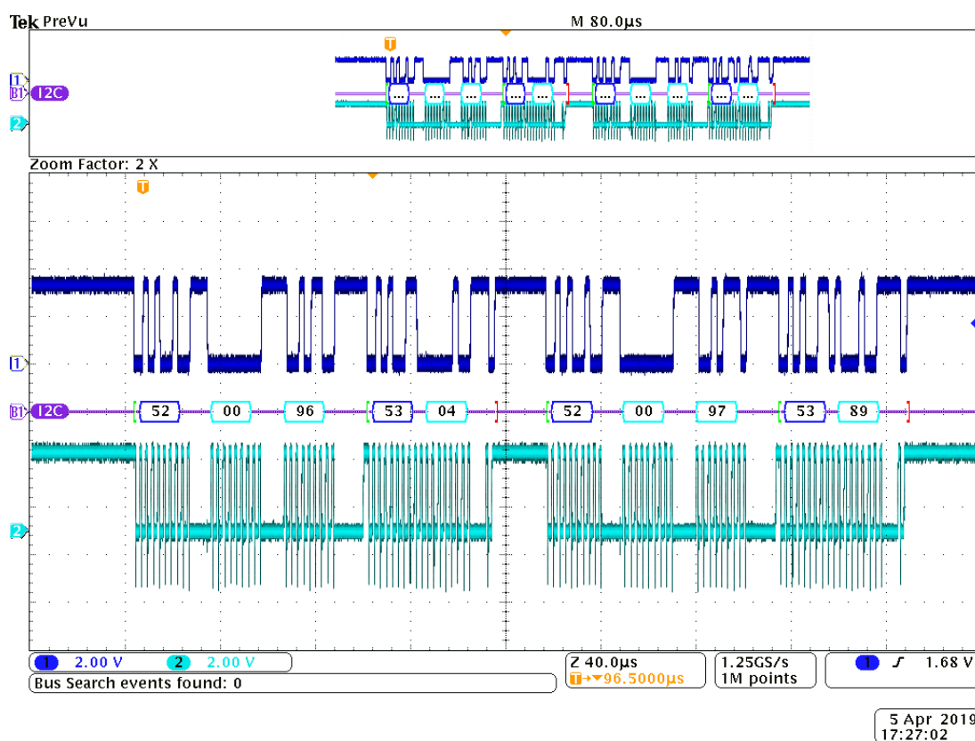
Obr. 9.1: Záznam z osciloskopu při rozcházení komunikace procesoru se senzorem VL53L1X po I 2 C sběrnici
