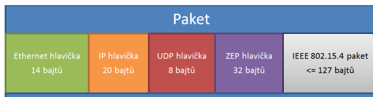
Obr. 5.1: Struktura paketu odeslaného z analyzátoru
