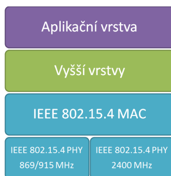
Obr. 1.2: Vrstvový model
