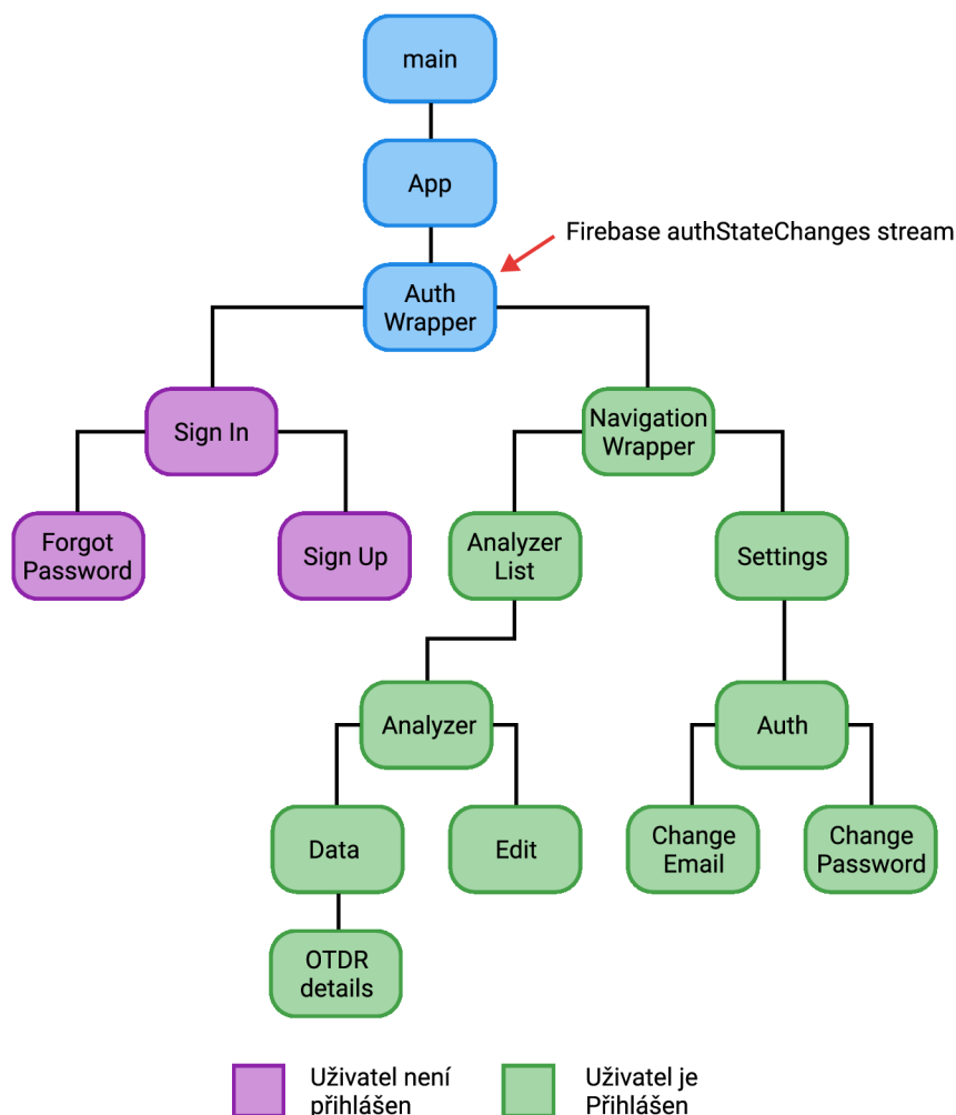
Obr. 7.1: Architektura aplikace.
