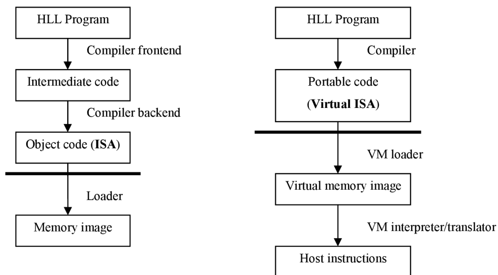
Obrázek 7: Srovnání běžného překladač (vlevo) s překladačem do přenositelného kódu (vpravo) [1] .
