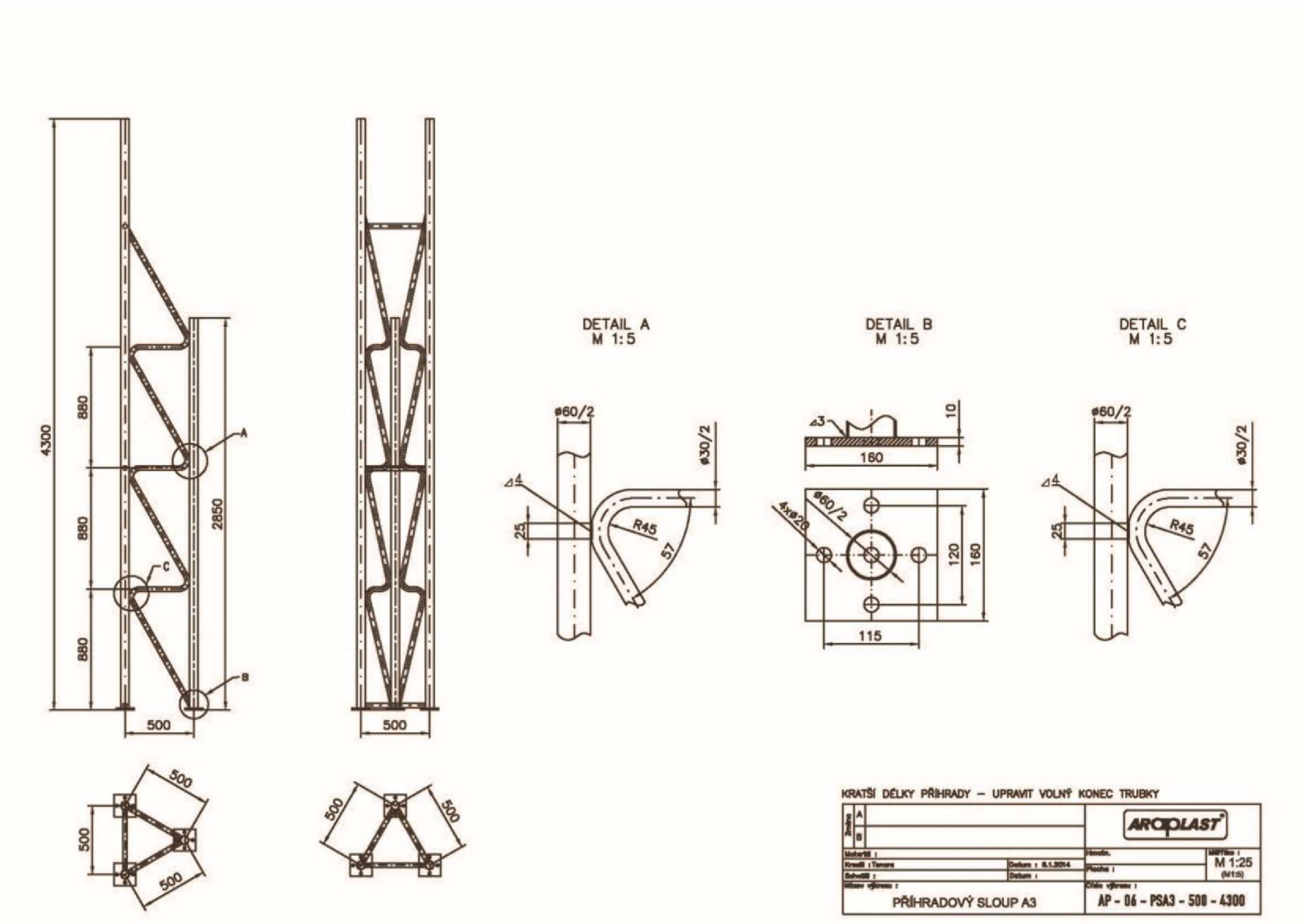
Příloha 2: Výkresová dokumentace nového typu příhradového nosníku rozměr 4300 mm
