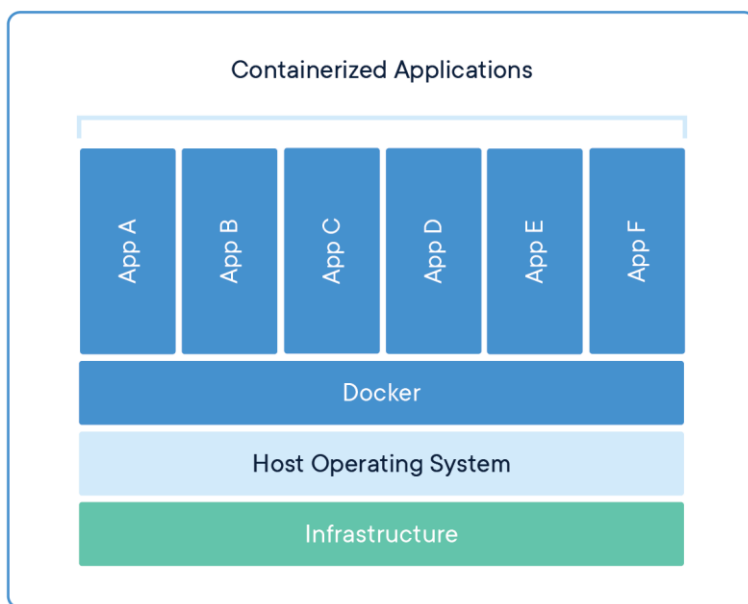
Obrázek 24 Docker
