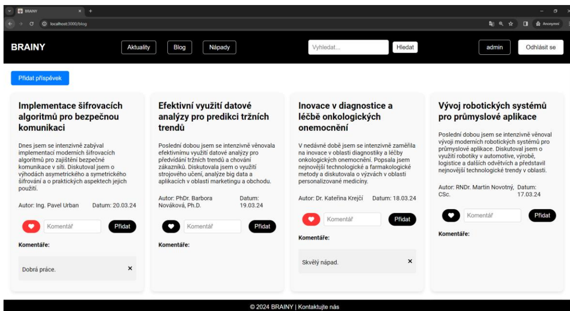
Obrázek 19 Blog React
