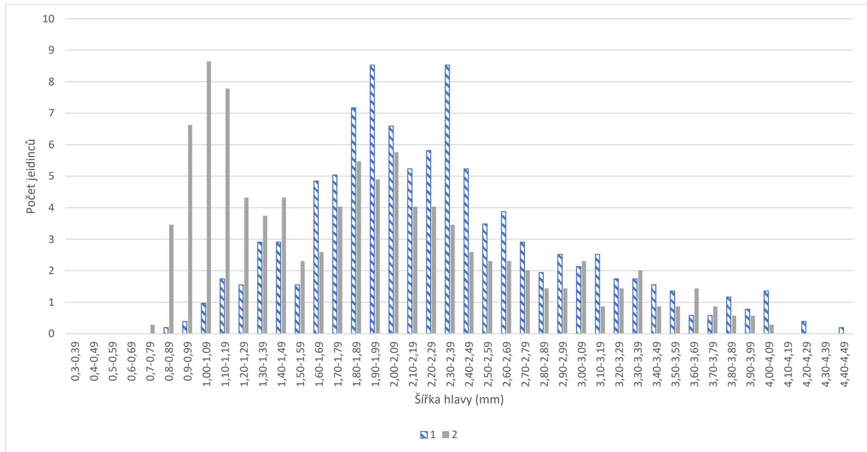
Příloha 2: Histogram šířky hlavy (mm) Atta sexdens v jednotlivých hrobečkách v odběru 25.1. - 8.2. 2023
