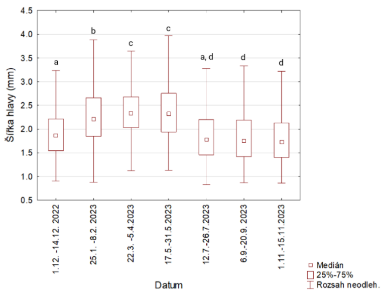
Graf 3.4: Porovnání šířky hlavy (mm) v hrobočku 1 v jednotlivých odběrech
