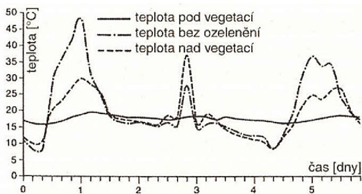
Graf 3.1 - Průběh teploty u ozeleněné střechy v hloubce substrátu 10 cm ve srovnání s nezatravněnou střešní plochou a teplotou vzduchu za horkého letního dne [9, s. 11].
