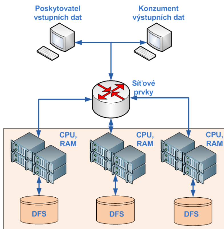
Obrázek 1.1: Použití několika výpočetních jednotek jako jeden superpočítač
