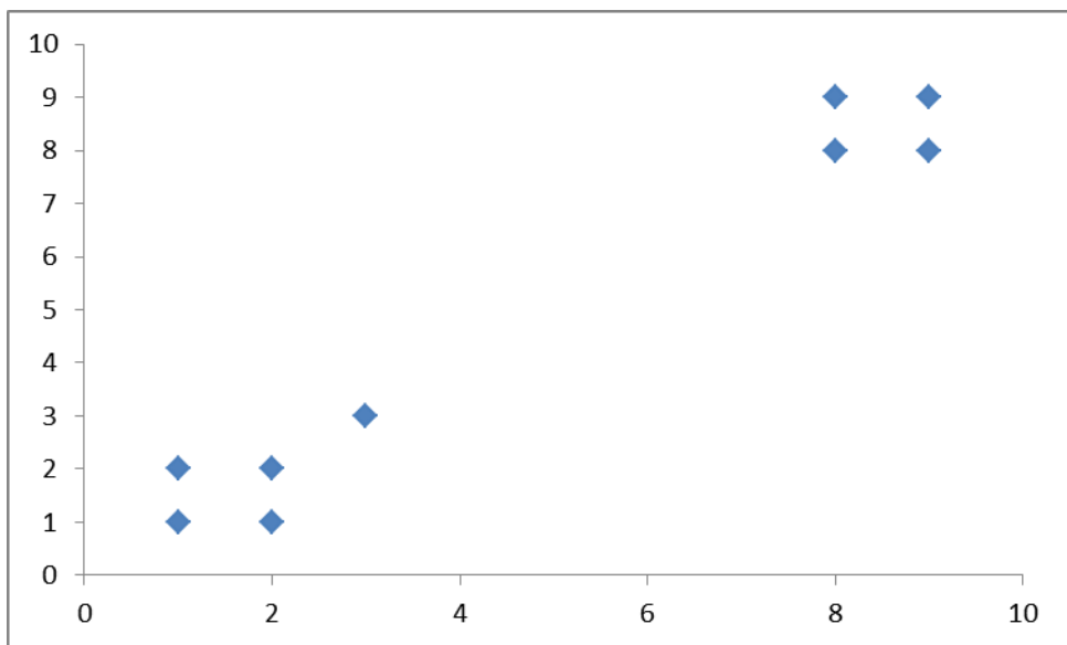
Obrázek 8.2: Grafické znázornění vektorů z Tabulka 8.2
