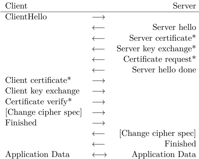
Tabuľka 2.1: Handshake priebeh [5]
