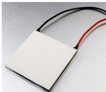
Obr. 5 – TEG/TEC článek 40 x 40mm [11]
