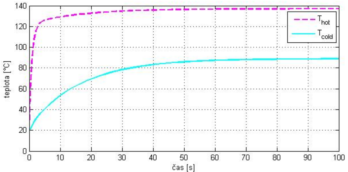
Obr. 23 – Průběh teplot uvnitř článku na počátku zahřívání
