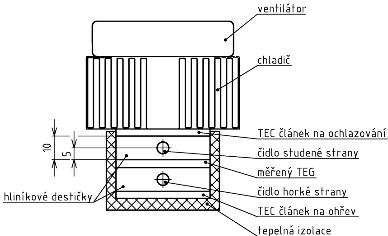
Obr. 26 – Měřicí soustava
