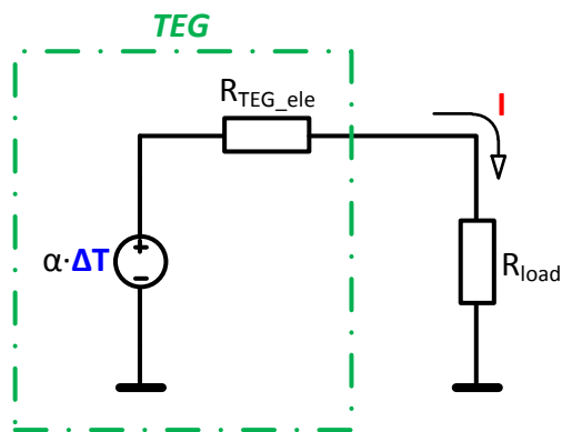
Obr. 20 – Elektrická část termočlánu
