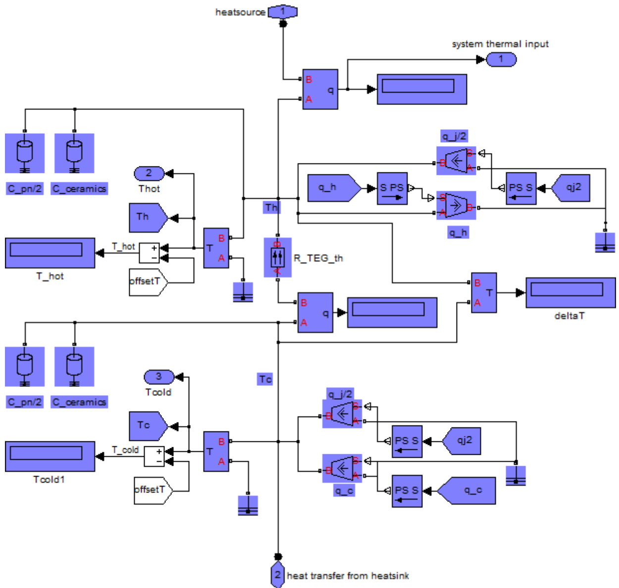
Obr. A3 – Tepelná větva v subsystemu TEG_th
