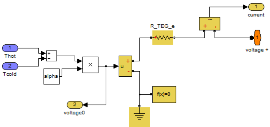
Obr. A5 – Subsystém TEG_e
