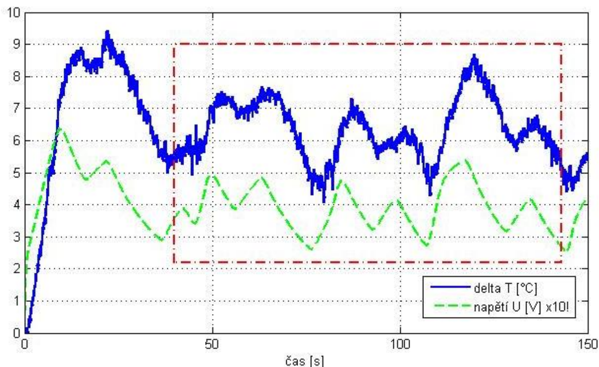
Obr. 28 – Příklad výběru dat a určení hodnot
