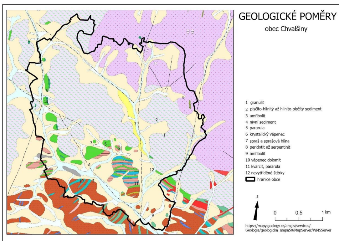
Obrázek 3.2: Geologické poměry v obci Chvalšiny
