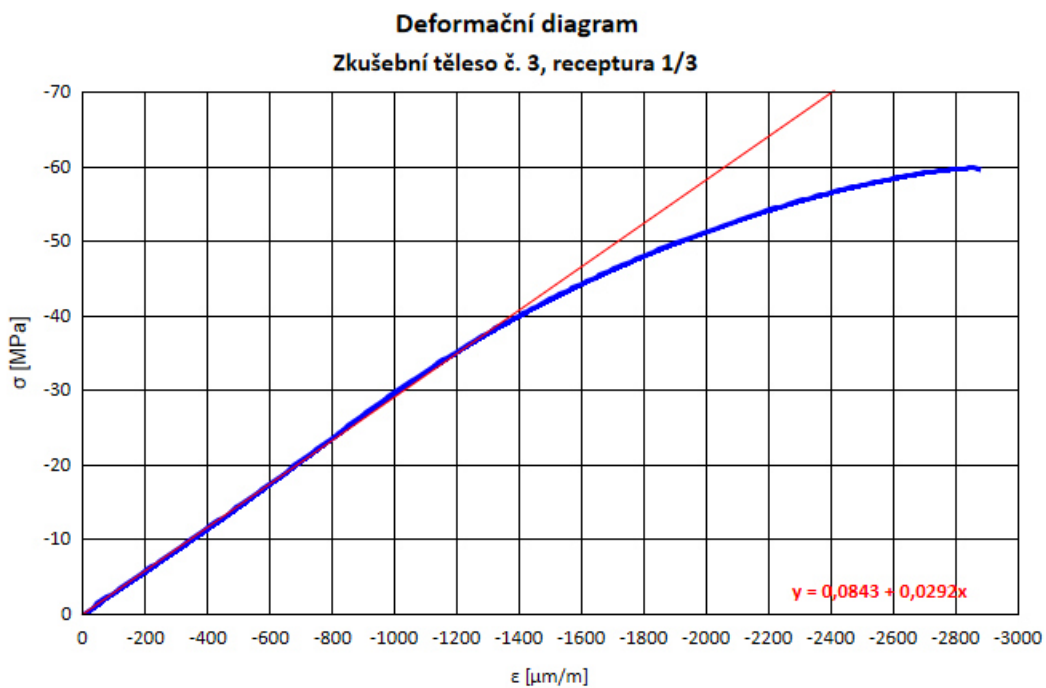
Obr. 8 Deformační diagram; zkušební těleso č. 3, receptura betonu 1/3
