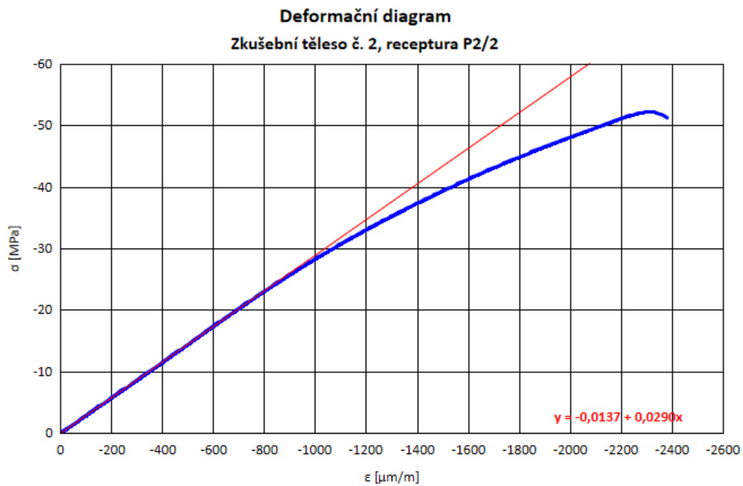
Obr. 12 Deformační diagram; zkušební těleso č. 2, receptura betonu P2/2
