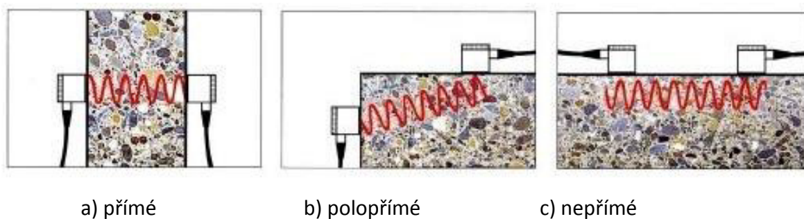
Obr. 5 Typy prozvučování měřeného objektu [14]
