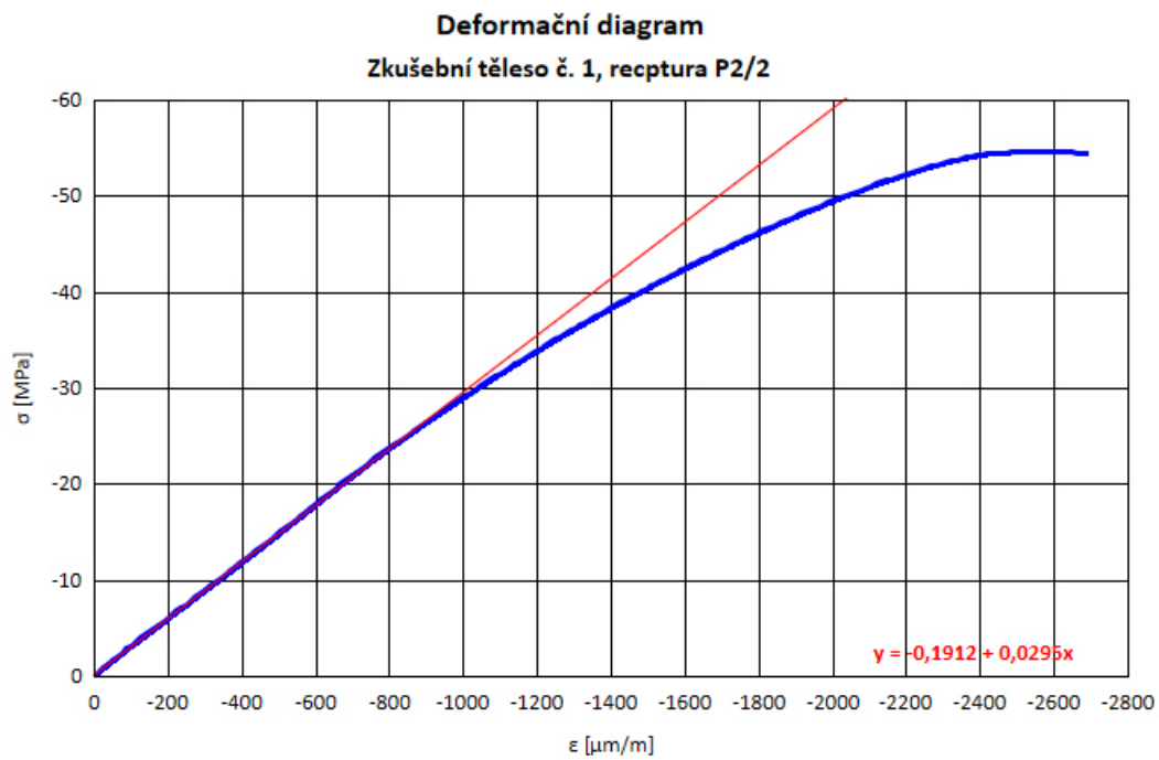
Obr. 11 Deformační diagram; zkušební těleso č. 1, receptura betonu P2/2
