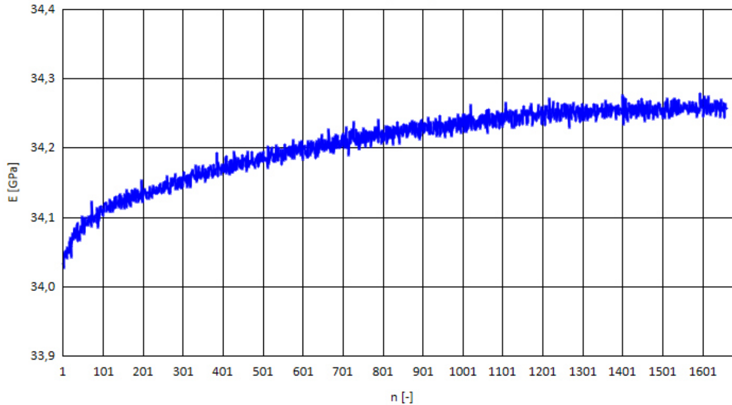
Obr. 4 Spojnicový graf závislosti statického modulu pružnosti v tlaku na počtu zatěžovacích cyklů; zkušební těleso č. 5, receptura betonu 2/3
