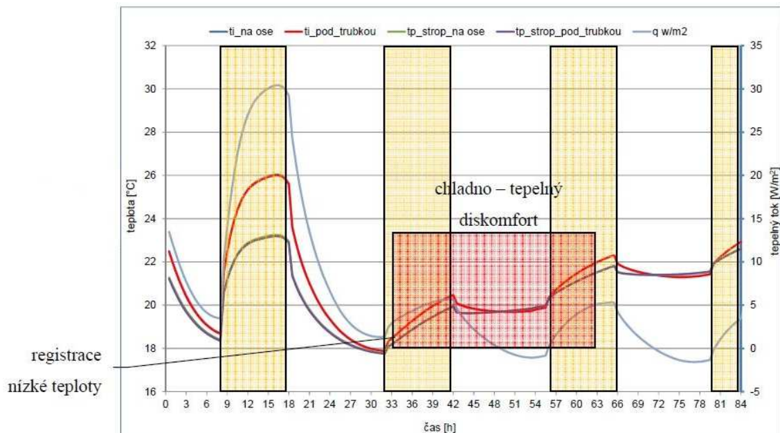
Obr. 7 Odezva systému [12]
