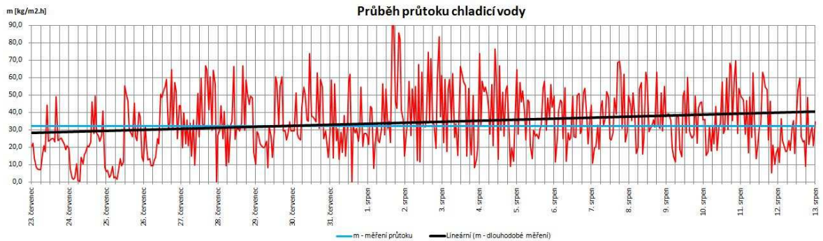
Obr. 42 Měrný průtok chladicí vody [Autor]
