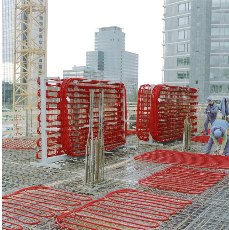
Obr. 20 Montáž tepelně aktivované stropní konstrukce [15]
