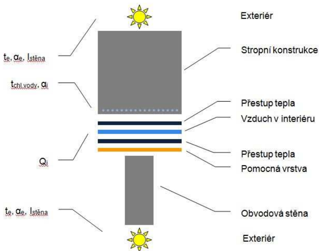
Obr. 45 Model – fyzikální představa [Autor]
