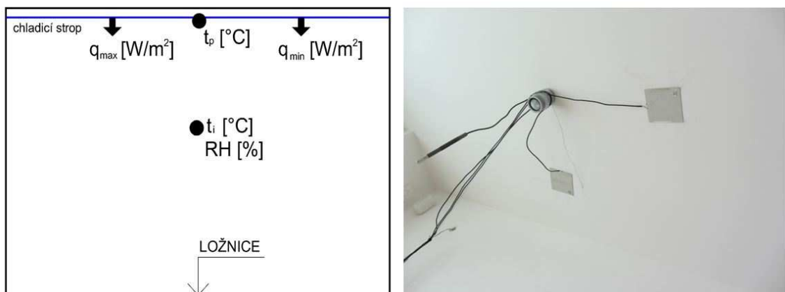
Obr. 31 Osazení měřicích čidel v ložnici [Autor]
