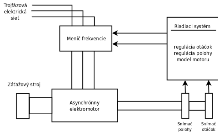
Obrázok 2.4: Diagram pohybových komponent
