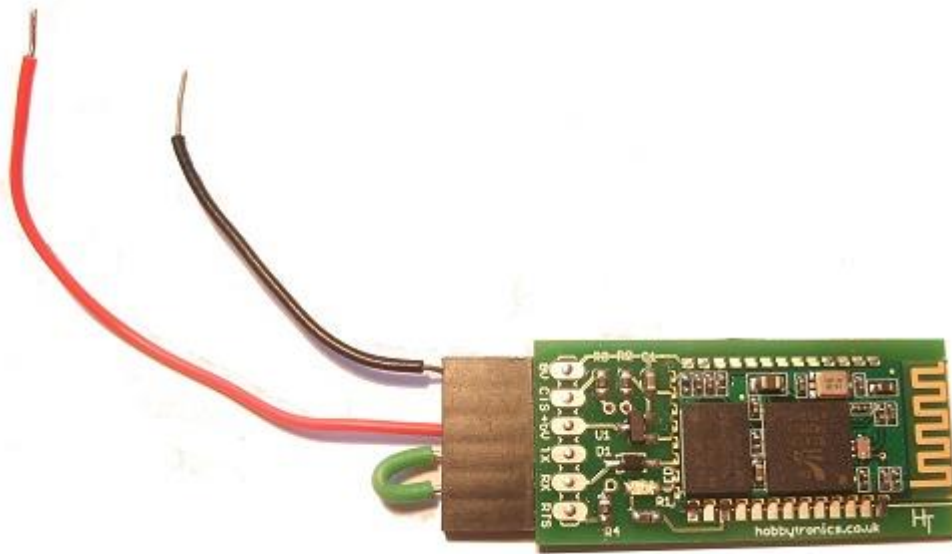
Obrázek 2.7 Bluetooth modul pro připojení [25]
