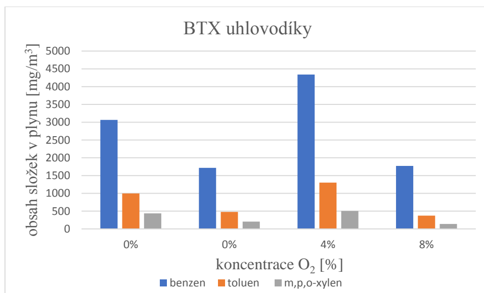
Obr. 6.6: Obsah BTX látek při různém obohacení
