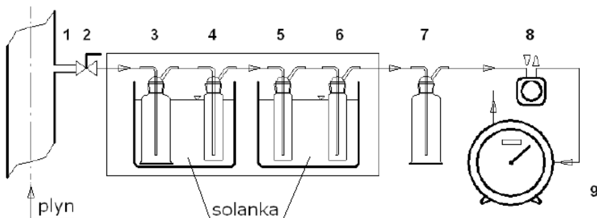
Obr. 5.6: Schéma upravené odběrové trati
