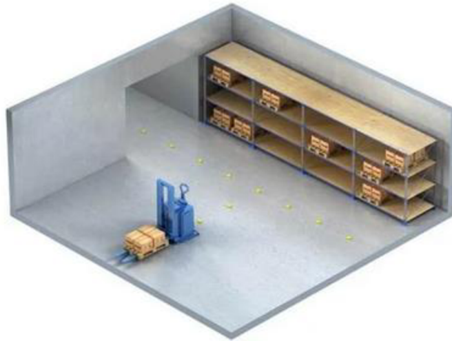
Obr. 3 Navigace pomocí magnetických značek
