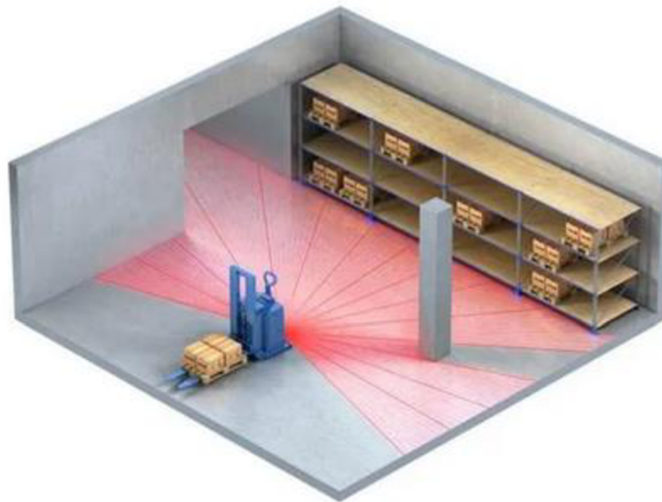
Obr. 9 Přirozená navigace
