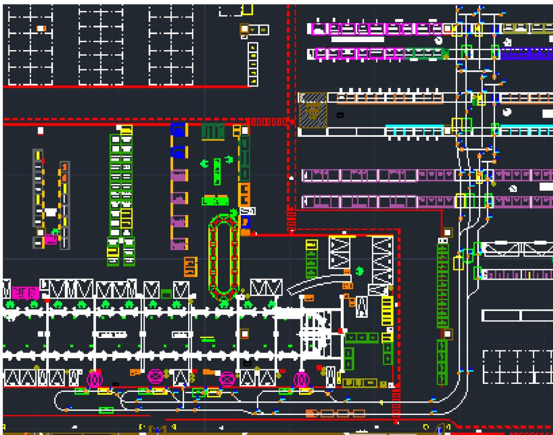
Zdroj: Interní dokumentace Obr. 15 Layout tras AGV
