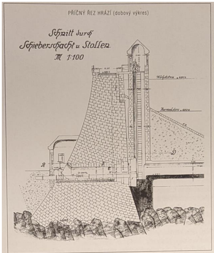
Obrázek 28 Příční řez hráze, Zdroj: (Broža, 2005)
