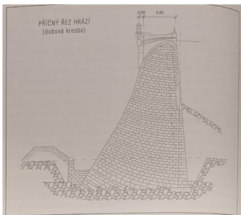
Obrázek 27 Příčný řez hrází, Zdroj:(Broža, 2005)
