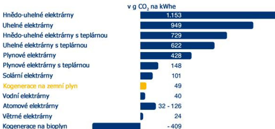
Obrázek 6 - produkce CO 2
