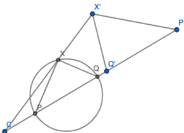
Obrázek 26: Inverze [10]
