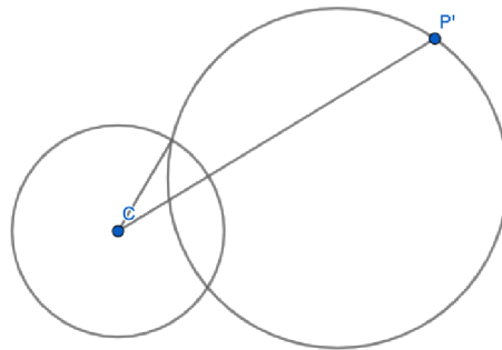
Obrázek 24: Inverze kružnic[10]
