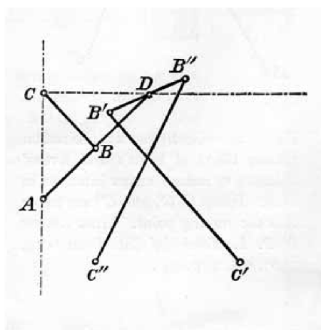
Obrázek 9: Návrh Chebysheva vynálezu[7]
