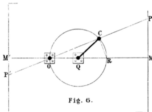
Obrázek 15: Geometrické zobrazení[1]
