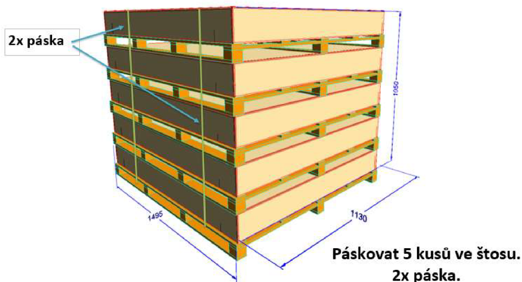
Obr. 2.8 Balící předpis výrobku KAR02394
