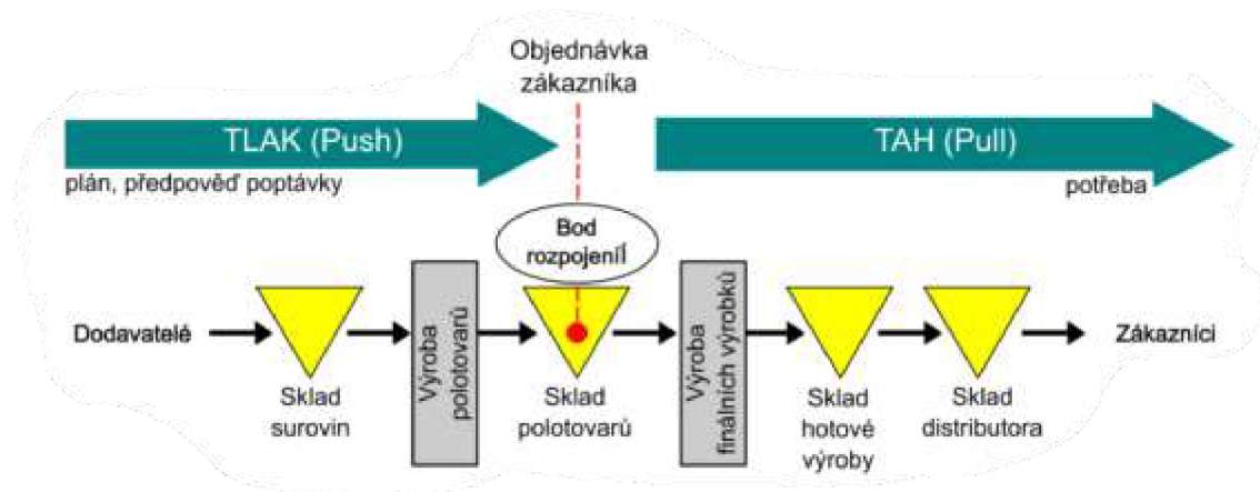
Obr. 1.1 Teorie bodu rozpojení
