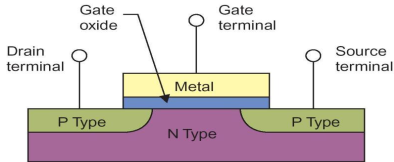
Obr. 2.5: Mosfet struktura – N-tyt
