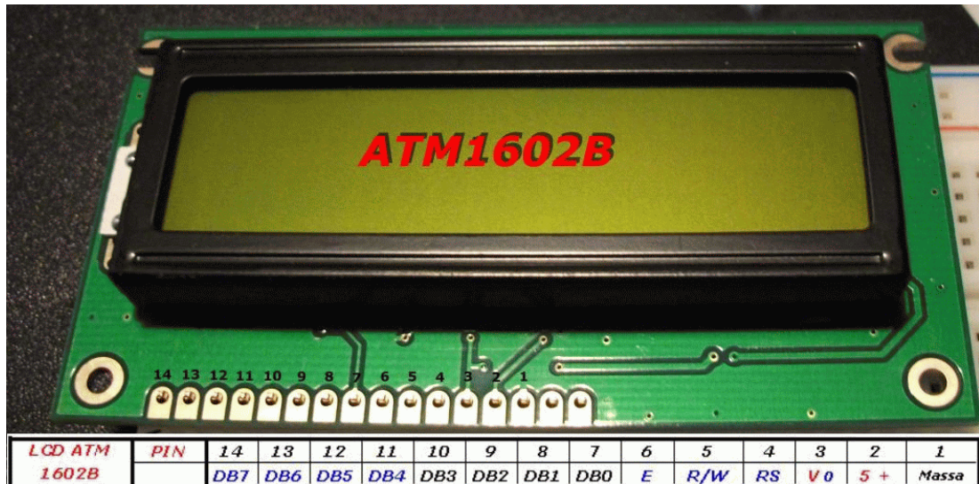
Obr. 2.13: Displej ATM1602B [14]
