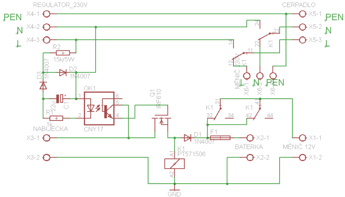
Obr. 4.9: Záložní zdroj
