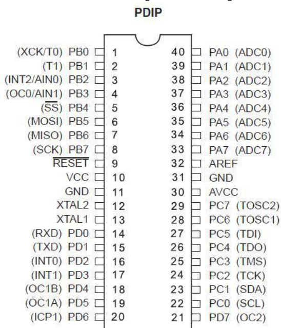
Obr. 2.2: Označení pinů [5] a pouzdro (DIL40) ATmega16
