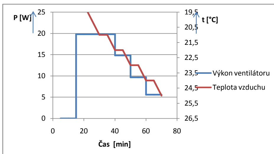
Obr. 4.7: Závislost výkonu ventilátoru a teploty vzduchu v místnosti na čase
