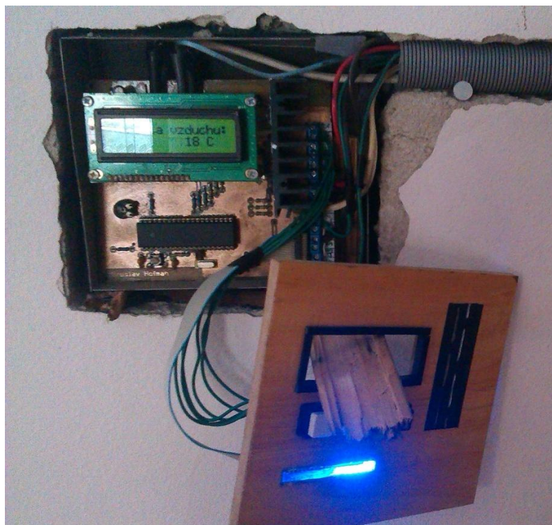
Obr. 4.3: Automatický regulátor
