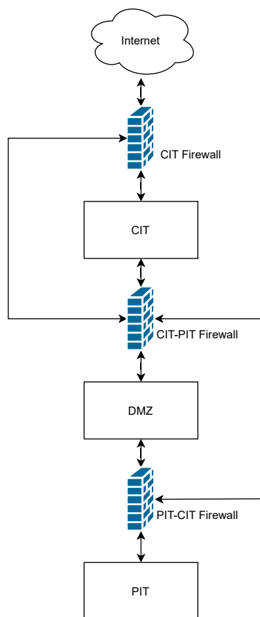
Obrázek 3.1: Schéma sítě
