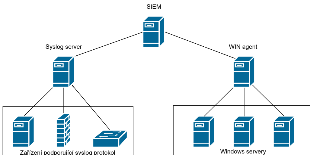
Obrázek 3.2: Architektura logování
