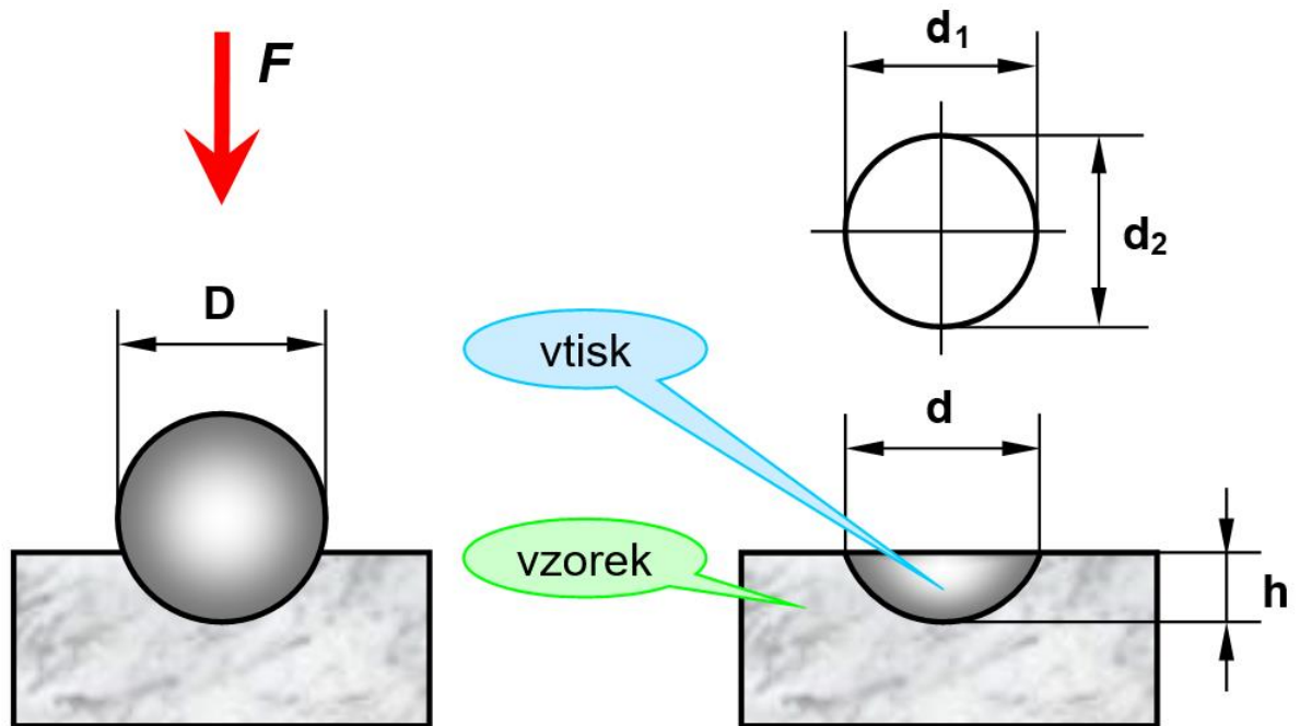
Obrázek 20: Schéma zkoušky tvrdosti podle Brinella (Zdroj [16])
