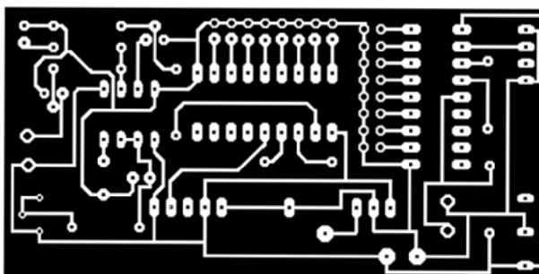
Obr. 25 návrh DPS-pager
