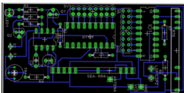
Obr. 24 osazovací plán-pager
