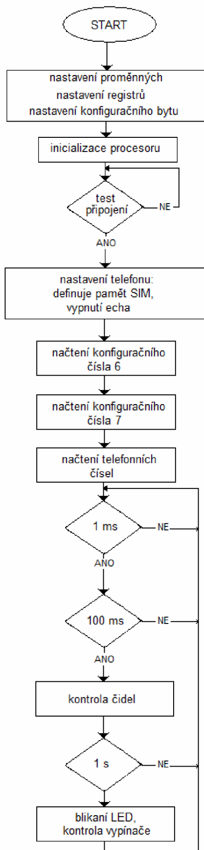
Obr. 20 vývojový diagram
