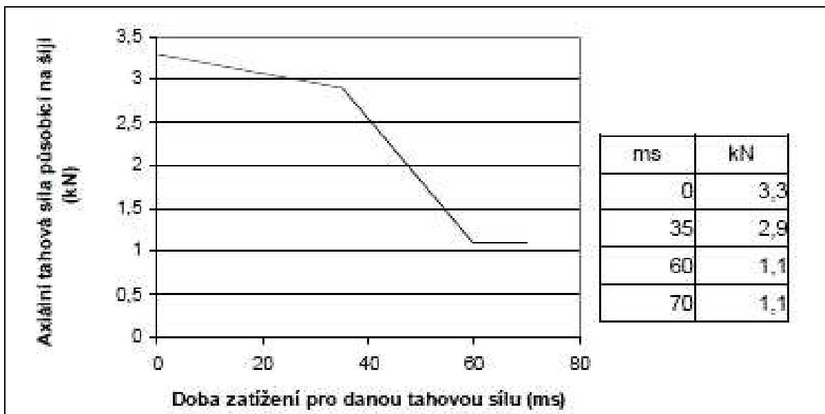
Obr. č. 36 Biomechanické kritérium tahu působícího na šiji při čelním nárazu do deformovatelné bariéry (převzato z [20])
