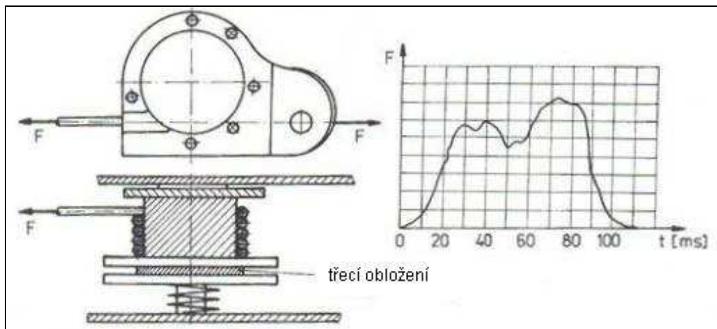
Obr. č. 24 Cívka s třecím obložním a graf průběhu síly působící na hrudník cestujícího při nárazu
