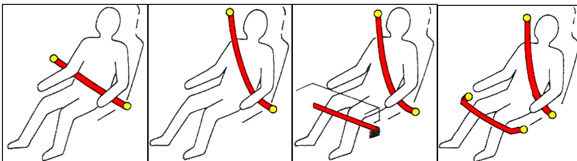
Obr. č. 9 Dvoubodový bezpečnostní pás: břišní, diagonální, diagonální s kolenní opěrkou, ramenní a kolenní ( zdroj [3])
