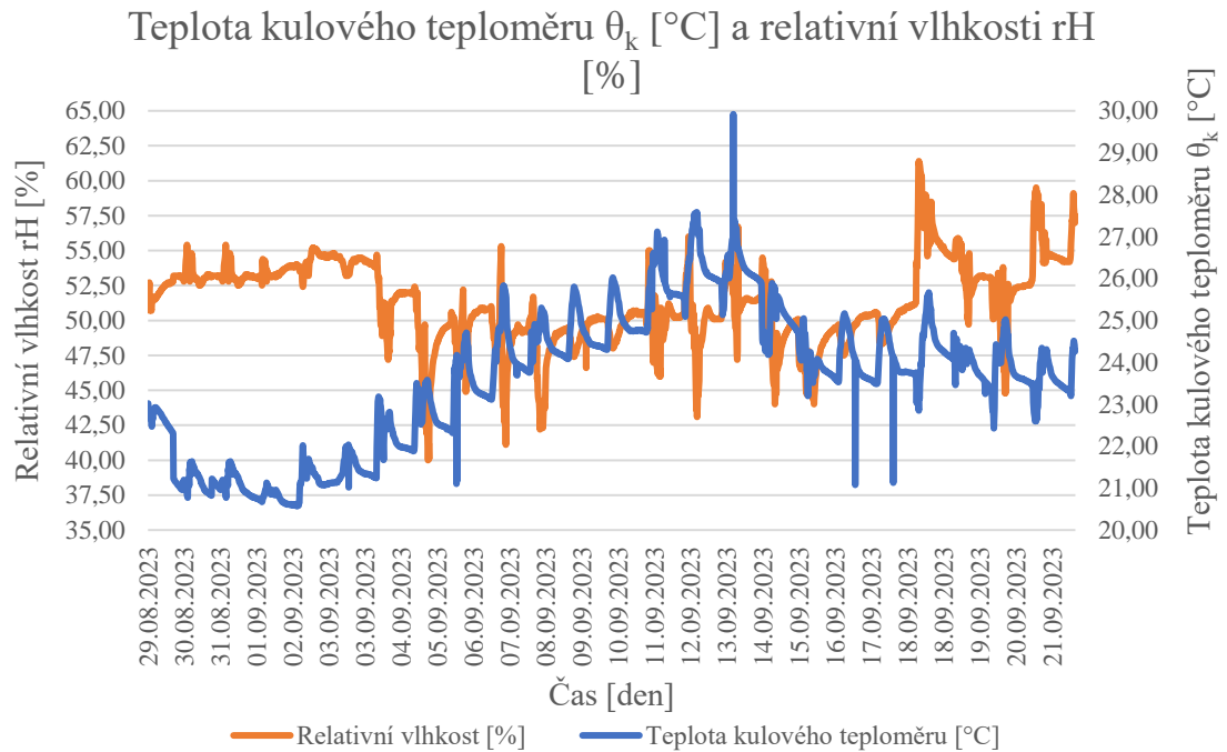
Graf 32.: Průběh měřené relativní vlhkosti rH [%] a teploty kulového teploměru \theta_k [°C] posuzované denní místnosti [vytvořeno autorkou]
