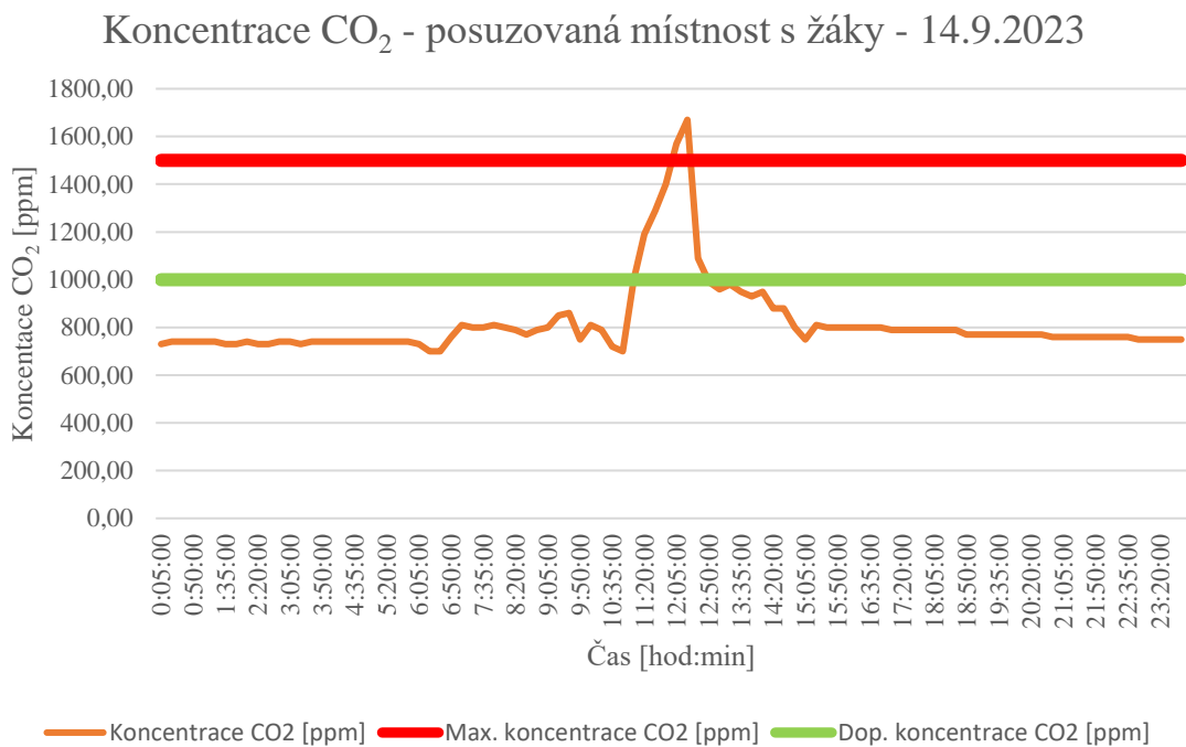
Graf 37.: Průběh koncentrace CO 2 v závislosti na počtu osob s porovnáním maximální a doporučené úrovně [1] – denní místnost s osobami
