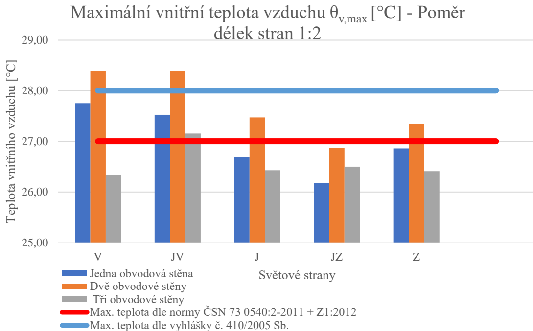
Graf 30.: Maximální vnitřní teplota vzduchu \theta_{v,max} [°C] získané z programu Simulace 2018 – Poměr délek stran 1:2 – navržené větrání
