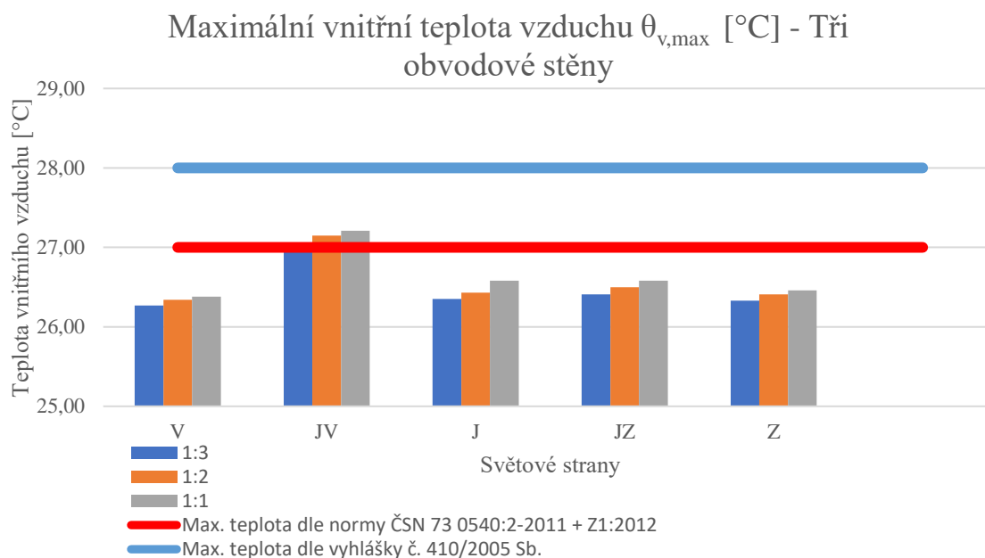
Graf 28.: Maximální vnitřní teplota vzduchu \theta_{v,max} [°C] získané z programu Simulace 2018 – Tři obvodové stěny – navržené větrání
