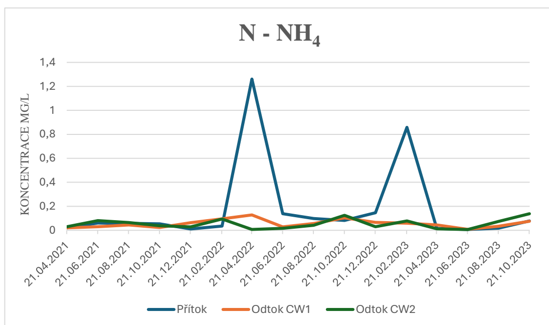
Graf 3: Koncentrace amoniakálního dusíku na přítoku, odtoku z horizontálního mokřadu (CW1) a odtoku z vertikálního mokřadu (CW2) v průběhu celého experimentu.
