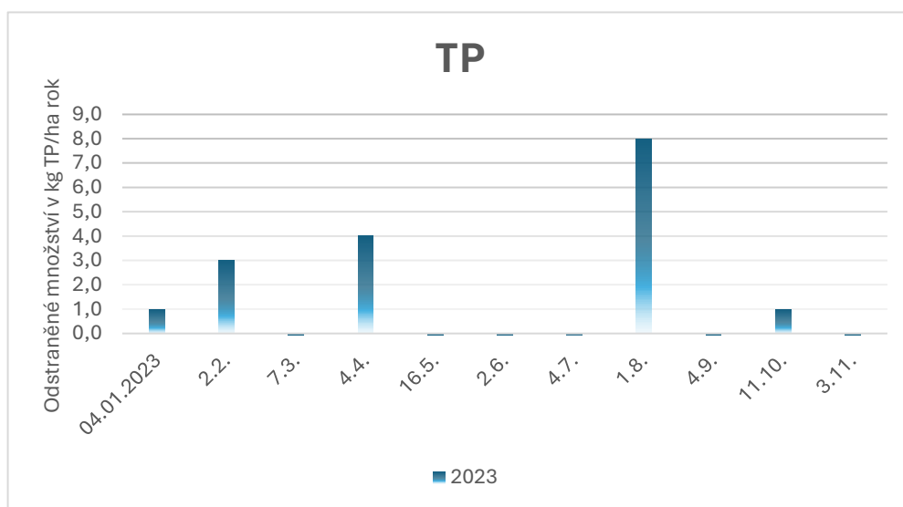
Graf č. 17: Odstraněné množství TP v umělém mokřadu Amálie v období od ledna do listopadu 2023.
