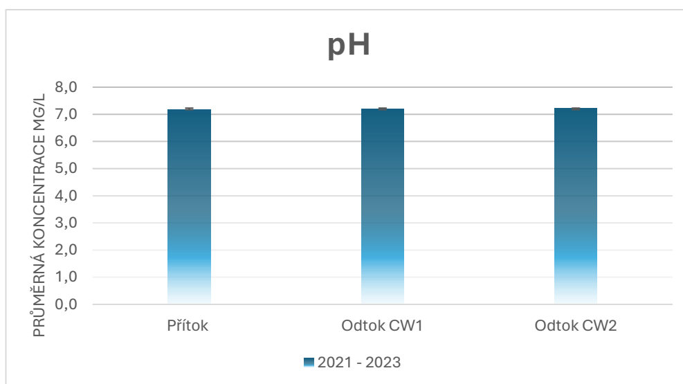
Graf 15: Výsledné hodnoty pH na přítoku, odtoku z horizontálního mokřadu (CW1) a odtoku z vertikálního mokřadu (CW2) v letech 2021-23.
