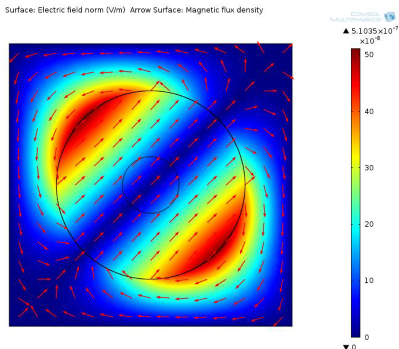
Obr. 3.5: Rozložení elektrického pole o frekvenci 1kHz
