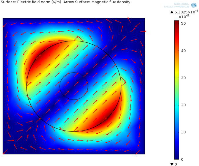
Obr. 3.3: Rozložení elektrického pole o frekvenci 1MHz
