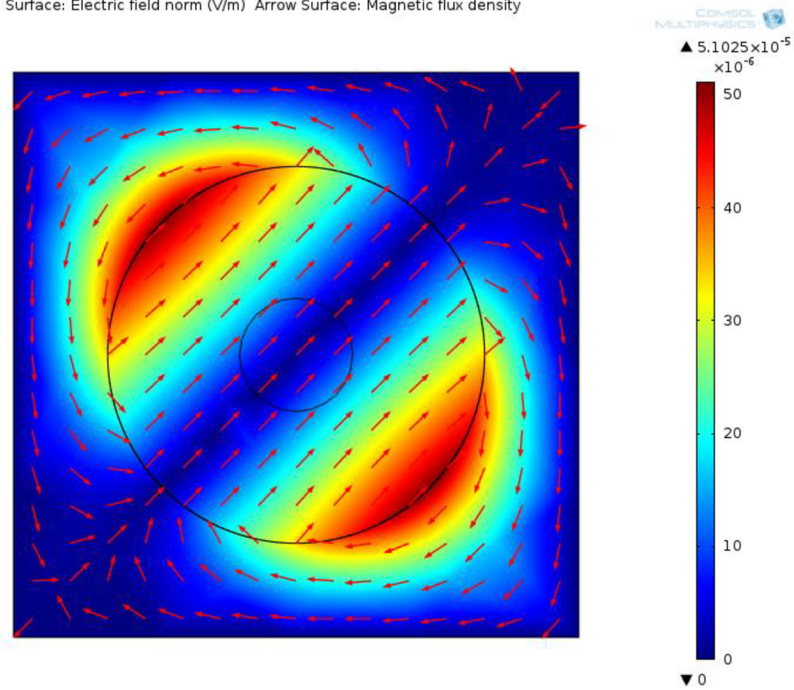
Obr. 3.2: Rozložení elektrického pole o frekvenci 100kHz
