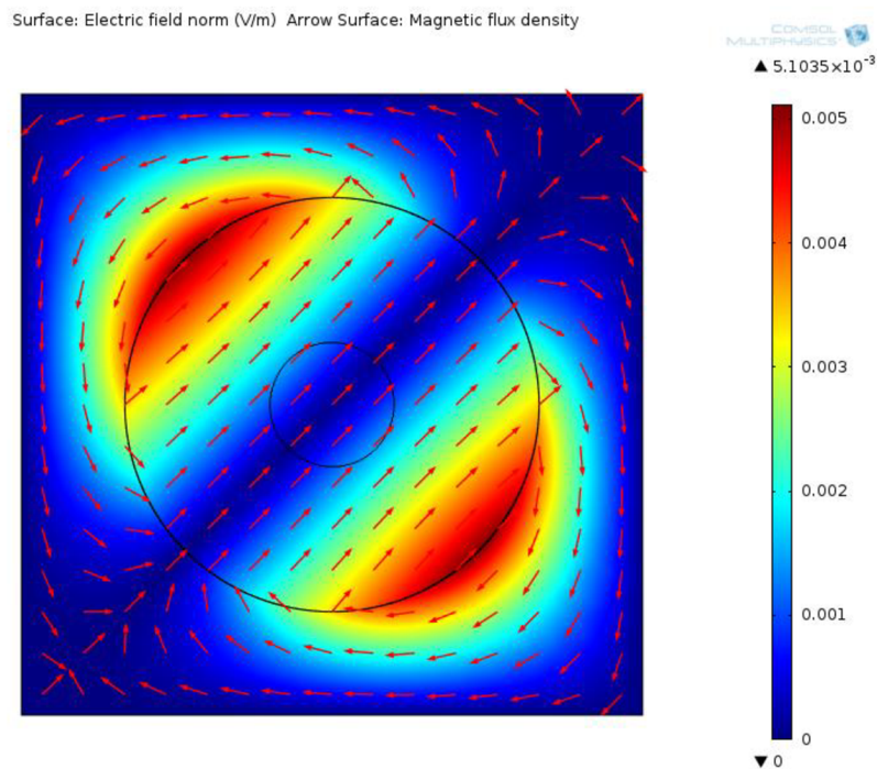
Obr. 3.8: Rozložení elektrického pole o frekvenci 10MHz
