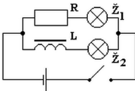
Obr. 1.12: Přechodný děj
