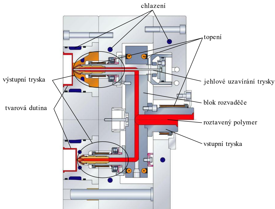
Obr. 9 Řez polovinou formy se zabudovaným systémem horkých vtoků [13]
