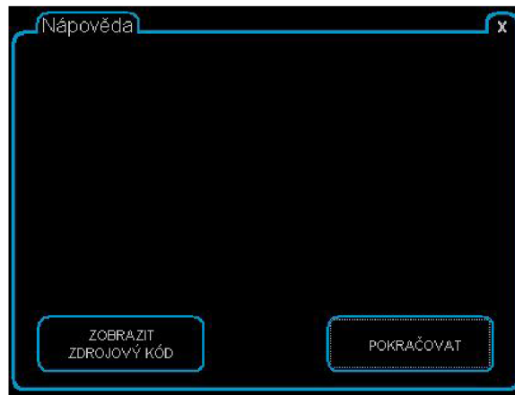
Obrázek 8.7: Nápověda
