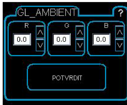
Obrázek 8.6: Ovládací panel
