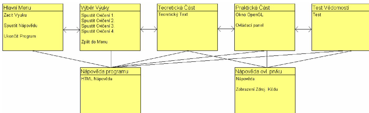
Obrázek 5.1: Návrh aplikace
