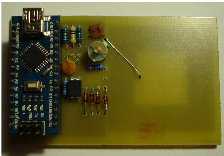
Obr. 2.7 - Vyrobený a osazený emulátor HF RFID tagu – přední strana
