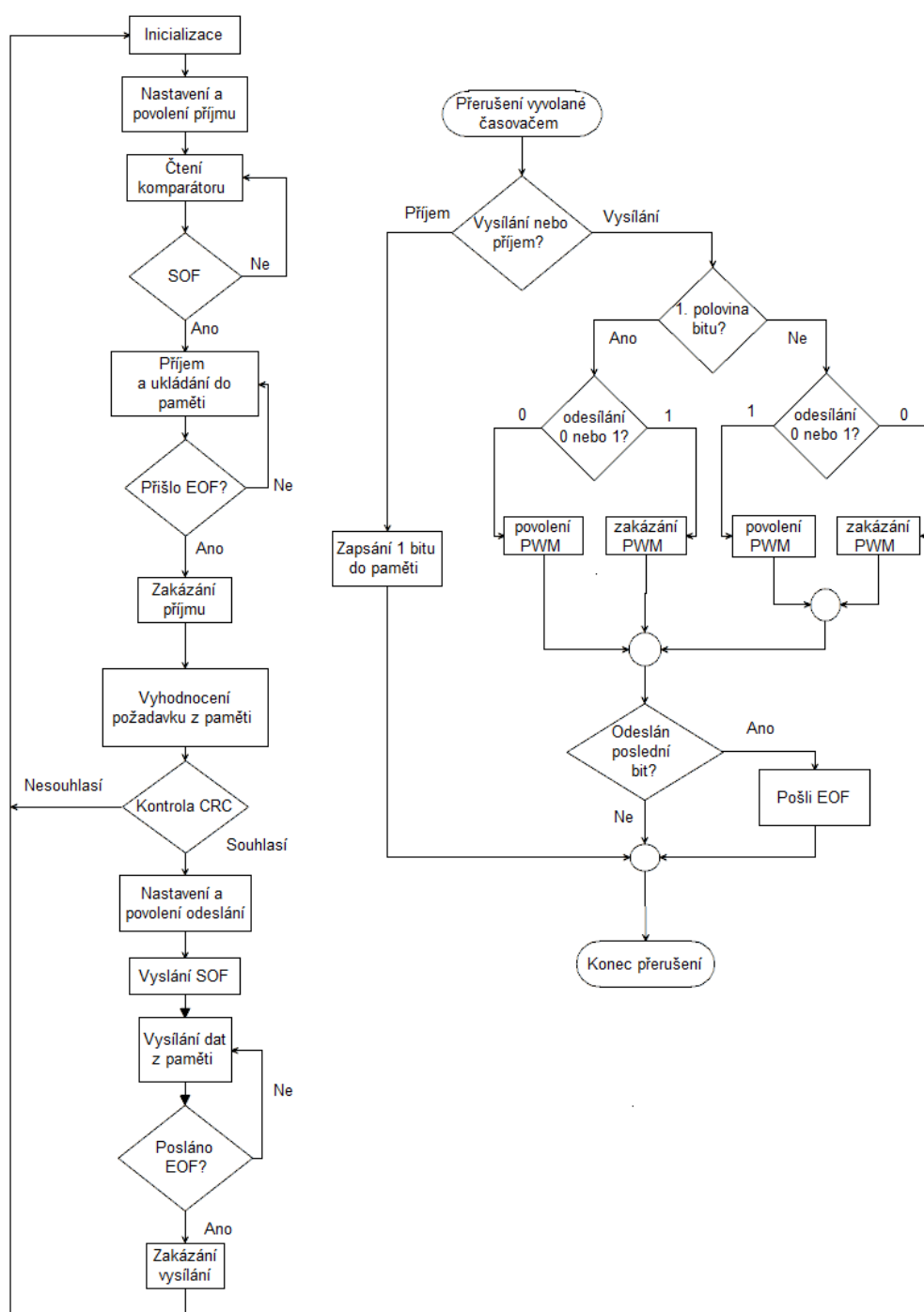
Obr. 3.13 – Vývojový diagram celého programu a diagram přerušení
