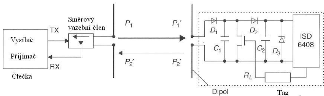
Obr. 1.11 – Princip RFID tagu využívající odrazovou metodu [6]
