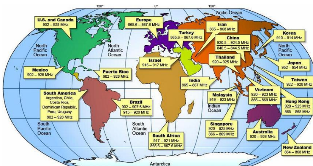
Obr. 1.2 – Pásmo UHF ve světě [5]
