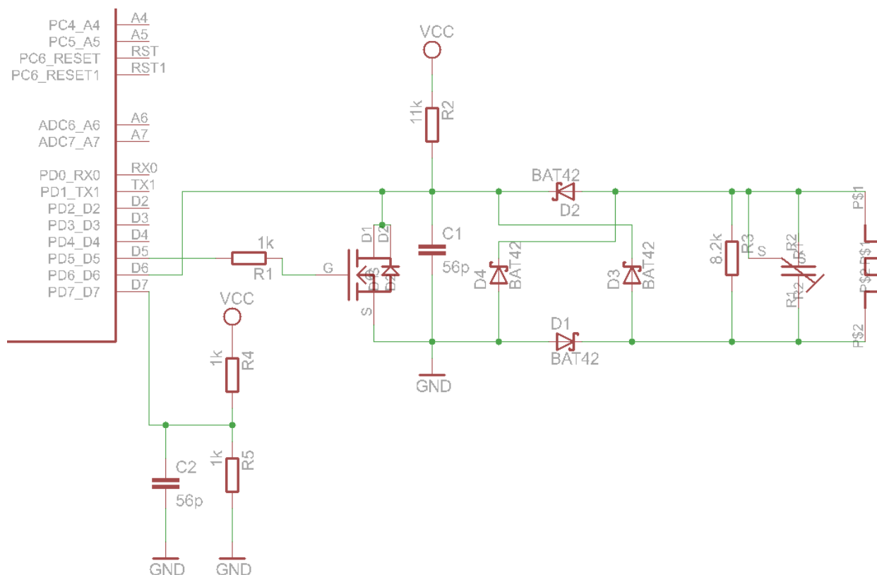
Obr. 2.4 – Analogová část emulátoru
