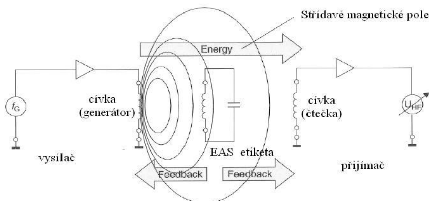
Obr. 1.7 – Princip radiofrekvenčního RFID tagu [6]
