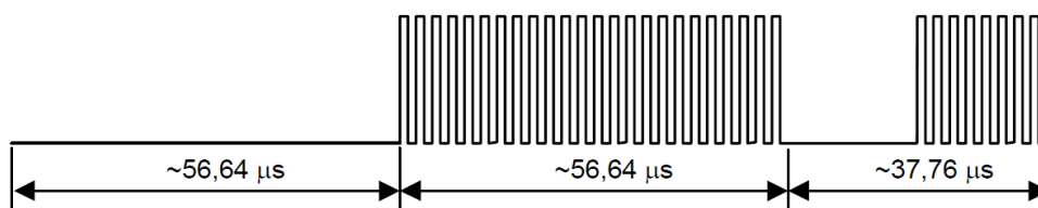
Obr. 3.10 – SOF s užitím jedné sub-nosné [22]
