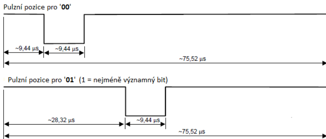
Obr. 3.3 – Typ kódování žádosti 1/4 [22]
