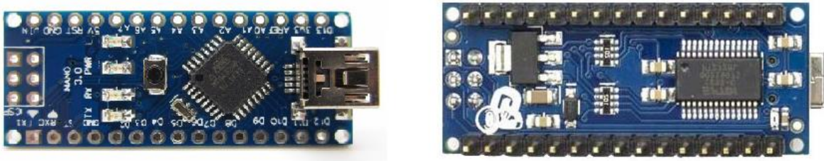
Obr. 2.5 – Platforma Arduino Nano – přední a zadní strana [23]
