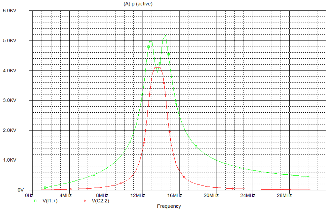
Obr. 2.3 – Přenosová charakteristika paralelních rezonančních obvodů čtečky a tagu
