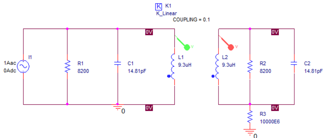
Obr. 2.2 - Vzájemná vazba dvou paralelních rezonančních obvodů
