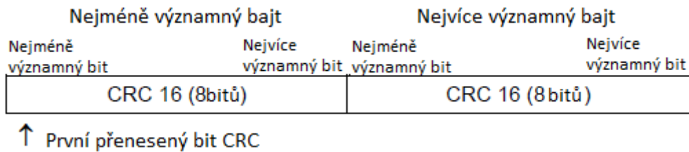
Obr. 3.2 – CRC kód [22]
