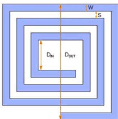
Obr. 2.1 – Planární čtvercová cívka a tabulka zvolených hodnot [20]
