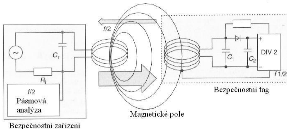
Obr. 1.9 – Princip RFID tagu využívající frekvenční dělič [6]
