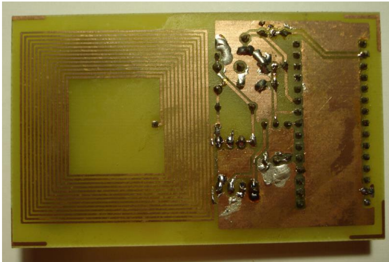
Obr. 2.6 - Vyrobený a osazený emulátor HF RFID tagu – zadní strana
