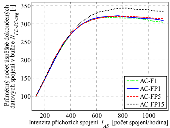
Obr. 6.39 Průměrný počet úspěšně dokončených datových spojení – převaha datových spojení
