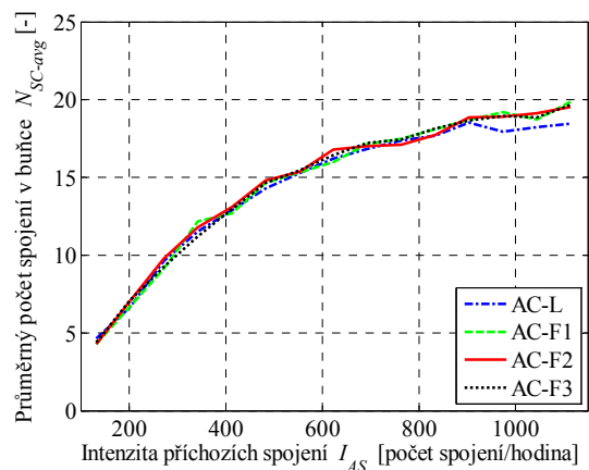
Obr. 4.45 Srovnání průměrného počtu spojení v buňce – převaha datových spojení
