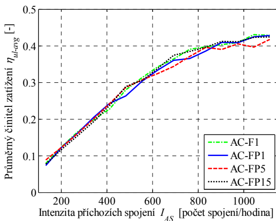
Obr. 6.30 Srovnání průměrných činitelů zatížení – převaha hlasových spojení
