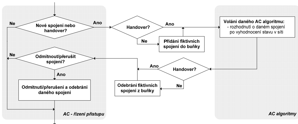
Obr. 5.2 Princip řízení přístupu pro AC-FP4
