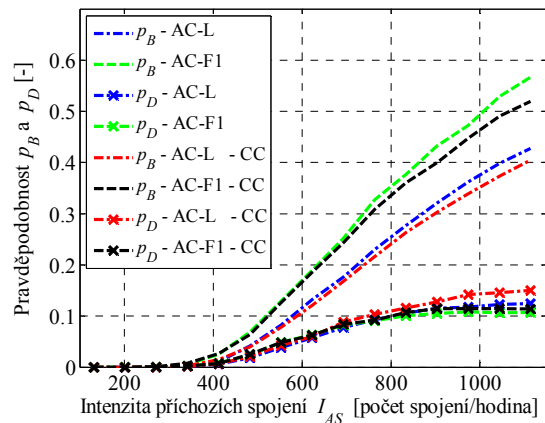
Obr. 4.10 Vliv řízení zahlčení sítě na datová spojení, průměrovací okno s délkou 20 sekund
