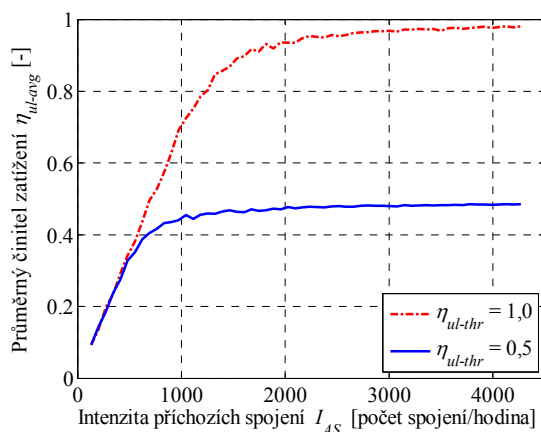
Obr. 2.6 Průměrný činitel zatížení \eta_{ul-avg} v buňce
