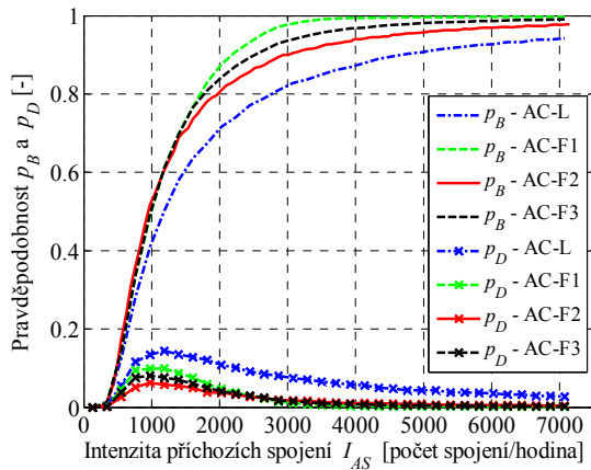
Obr. 4.58 Srovnání několika fuzzy algoritmů pro datová spojení – bez použití \Delta F_{thr}
