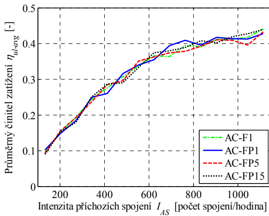
Obr. 6.20 Srovnání průměrných činitelů zatížení
