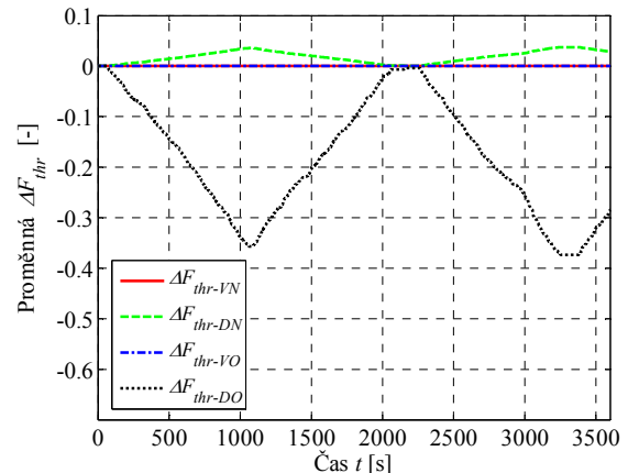
Obr. 6.55 Vývoj proměnných pro automatickou regulaci prahů pro AC-F1 R1
