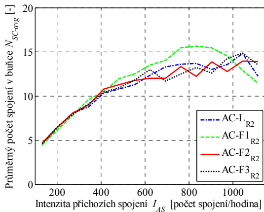
Obr. 6.64 Srovnání průměrného počtu spojení v buňce, \beta = 3
