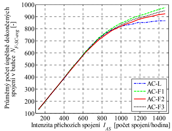
Obr. 4.33 Srovnání průměrného počtu úspěšně dokončených spojení v buňce
