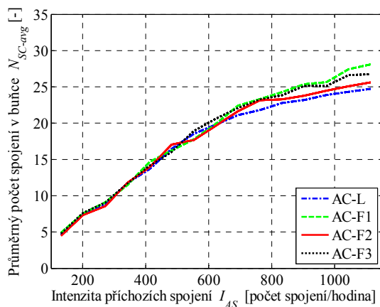
Obr. 4.44 Srovnání průměrného počtu spojení v buňce – převaha hlasových spojení
