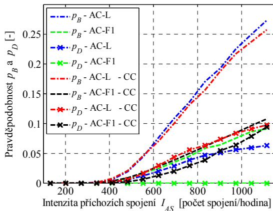
Obr. 4.9 Vliv řízení zahlčení sítě na hlasová spojení, průměrovací okno s délkou 20 sekund
