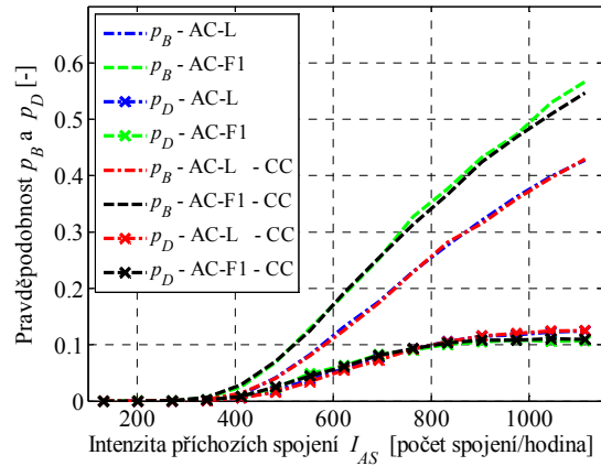
Obr. 4.8 Vliv řízení zahlčení sítě na datová spojení, průměrovací okno s délkou 30 sekund
