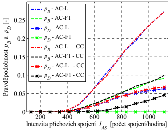
Obr. 4.7 Vliv řízení zahlčení sítě na hlasová spojení, průměrovací okno s délkou 30 sekund
