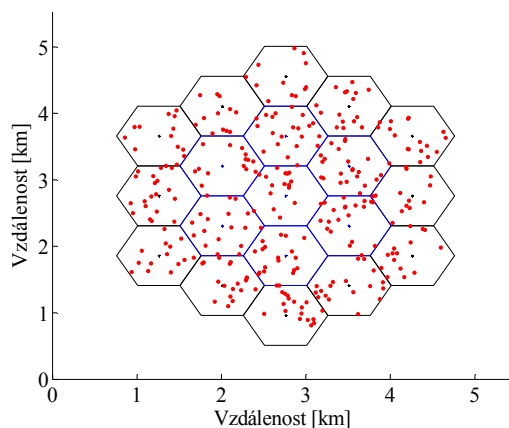
Obr. 2.2 Rozložení UEs v systému
