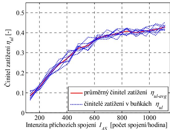
Obr. 4.96 Průběh činitelů zatížení \eta_{ul} pro AC-F1
