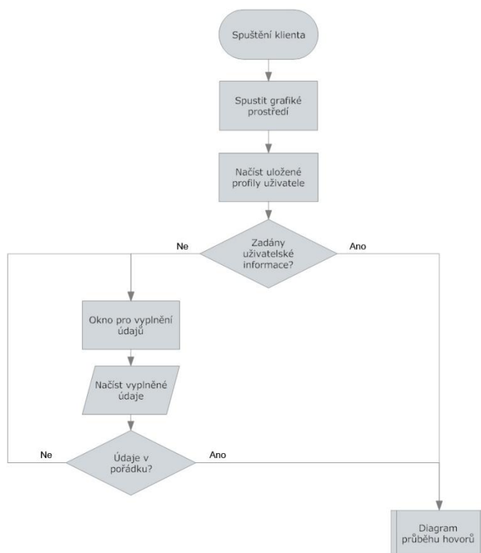
Obr. 4.1: Vývojový diagram při startu programu
