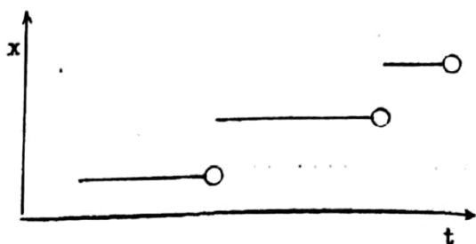
Obr. 3 Graf stochastického s diskrétním časem
