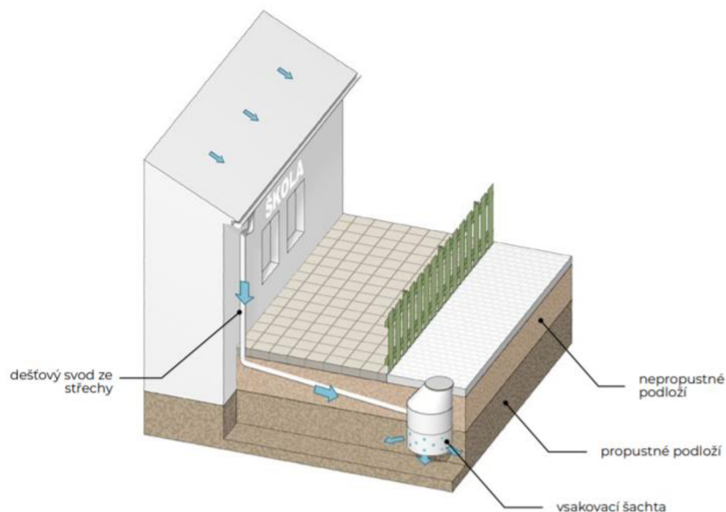
Obrázek 9 vsakovací šachta (Šýkorová a kol., 2021)
