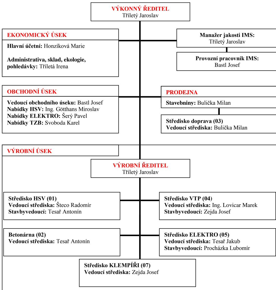
Obrázek 2: Organizační struktura [15]
