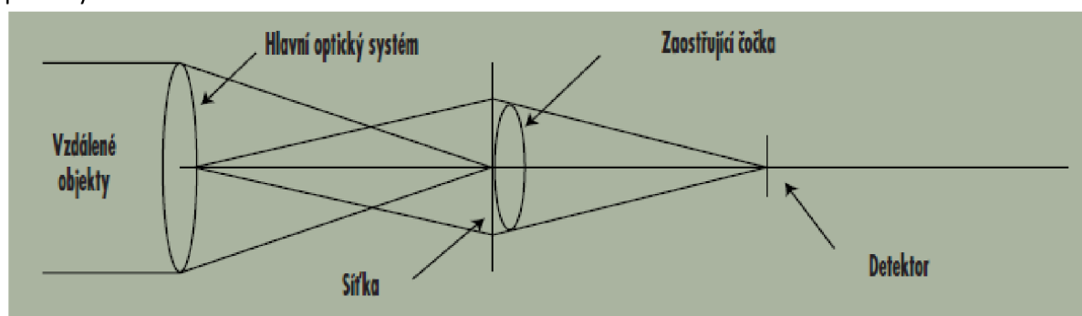
Obr.4: Infračervená optika naváděcího systému střely [1]
