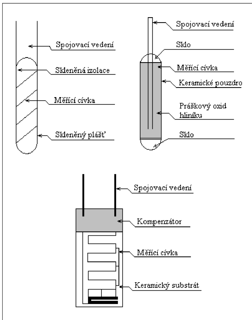
Obr. 3.2 Sklenné vinutí, keramické vinutí a odporové teploměry s tenkou vrstvou
