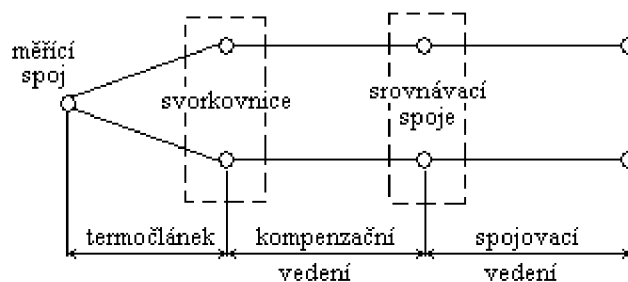
Obr. 3.5 Názvosloví termoelektrického teploměru
