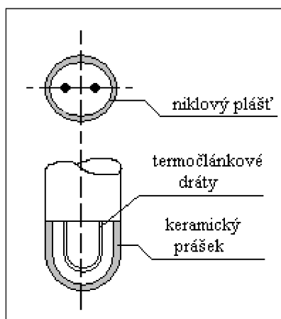
Obr. 3.7 Plášťový termočláňek
