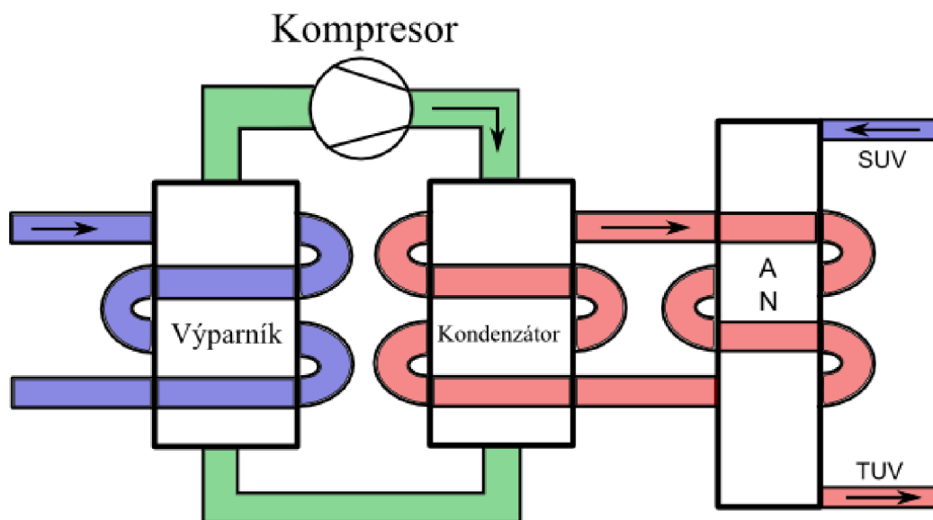
Obr. 6.2 Akumulační okruh
