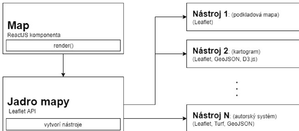
Obr. 6.1: Architektúra systému Geovisto a pridaný nástroj a jeho funkcie.
